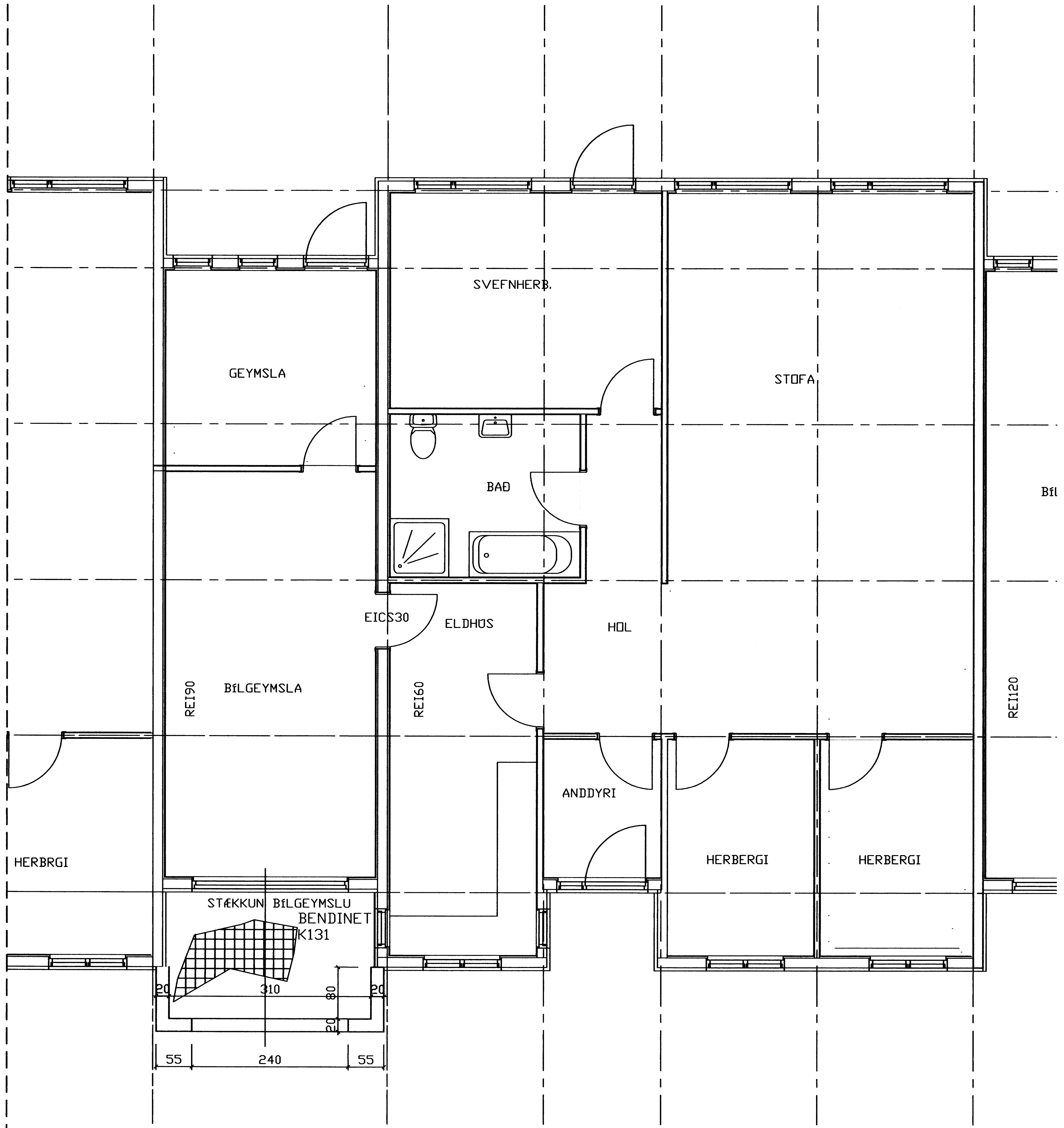
GRUNNMYND M=1:50
