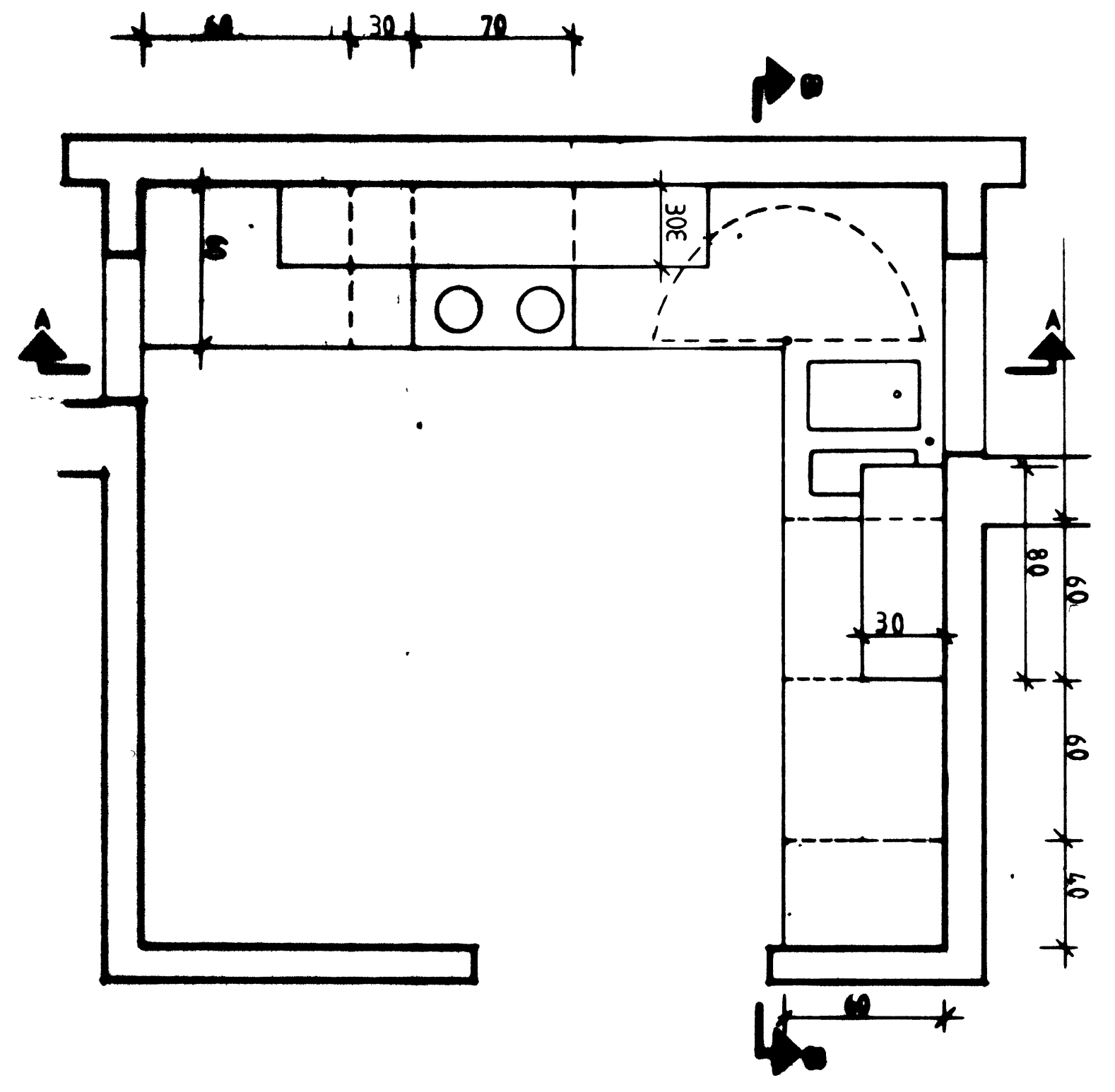
GRUNNMYND 120
