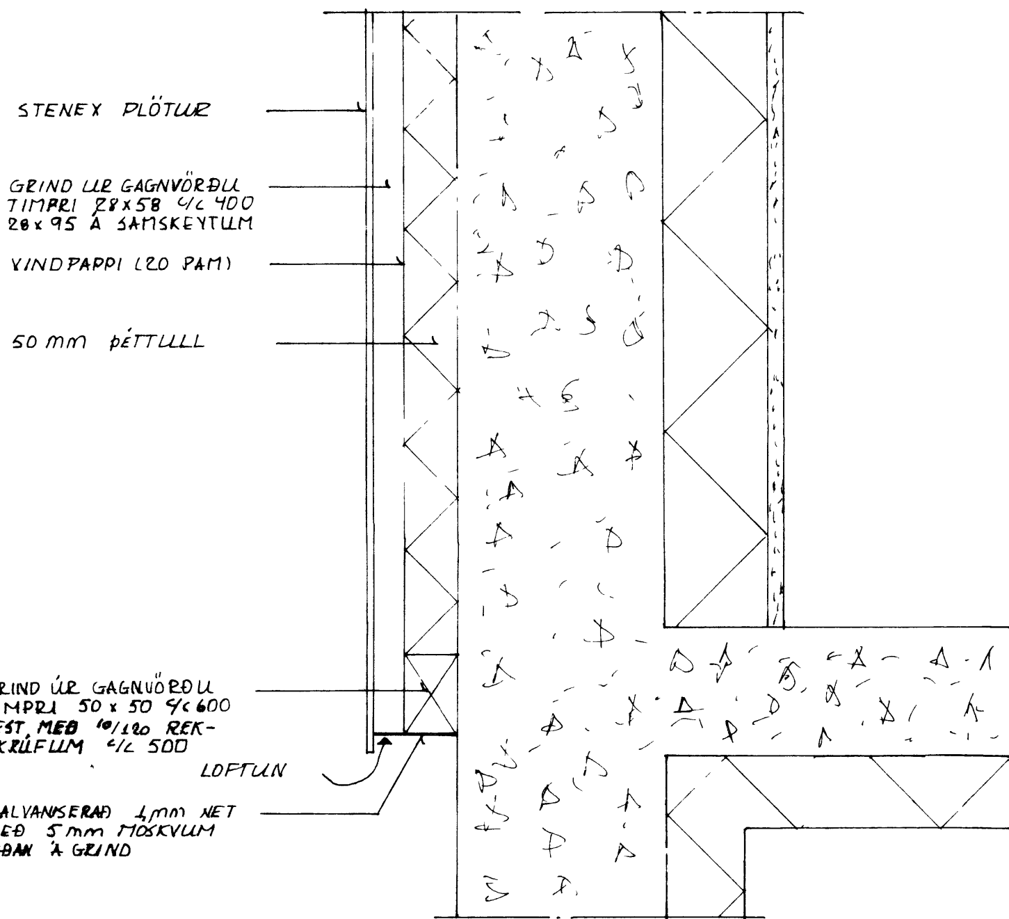
FRÁGANGUR AÐ NEÐAN LÖBRÉTT SNIÐ MKV 1.5
