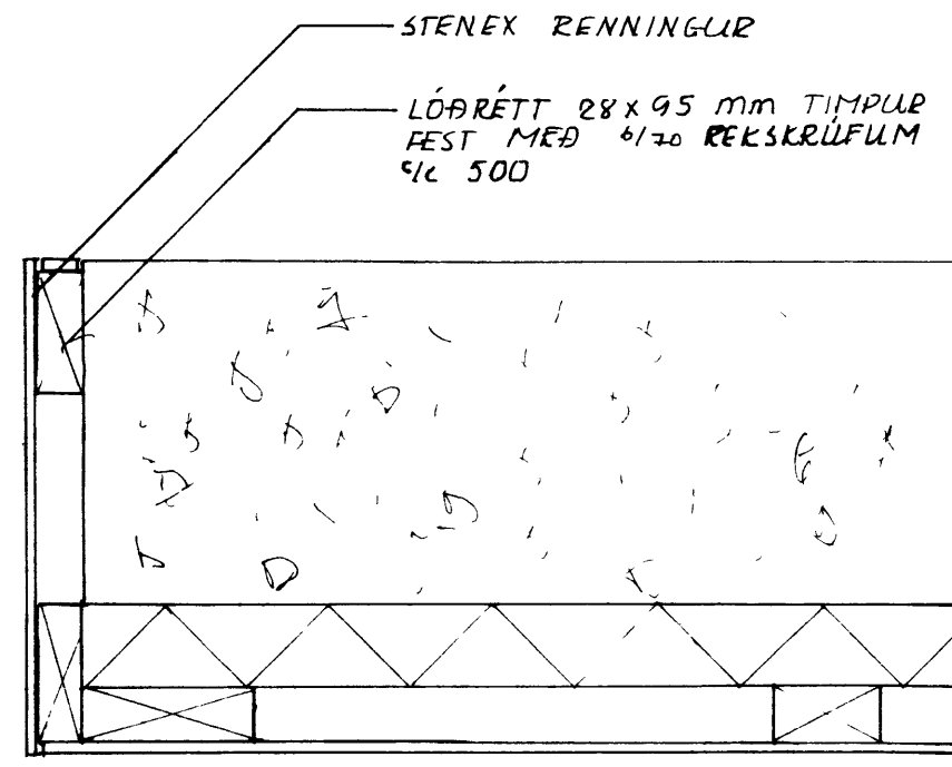
FRÁGANGUR Á ENDUM LÖBRÉTT SNIÐ MKV 1.5
