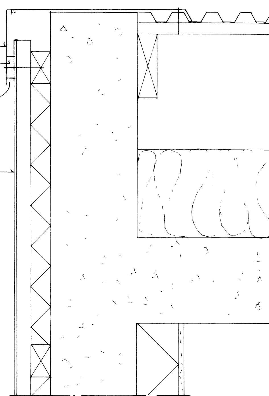
FRÁGANGUR AÐ OFAN LÖBRÉTT SNIÐ MKV 1.5
