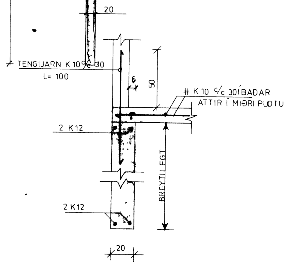
SNID A-A MKV 1:20
