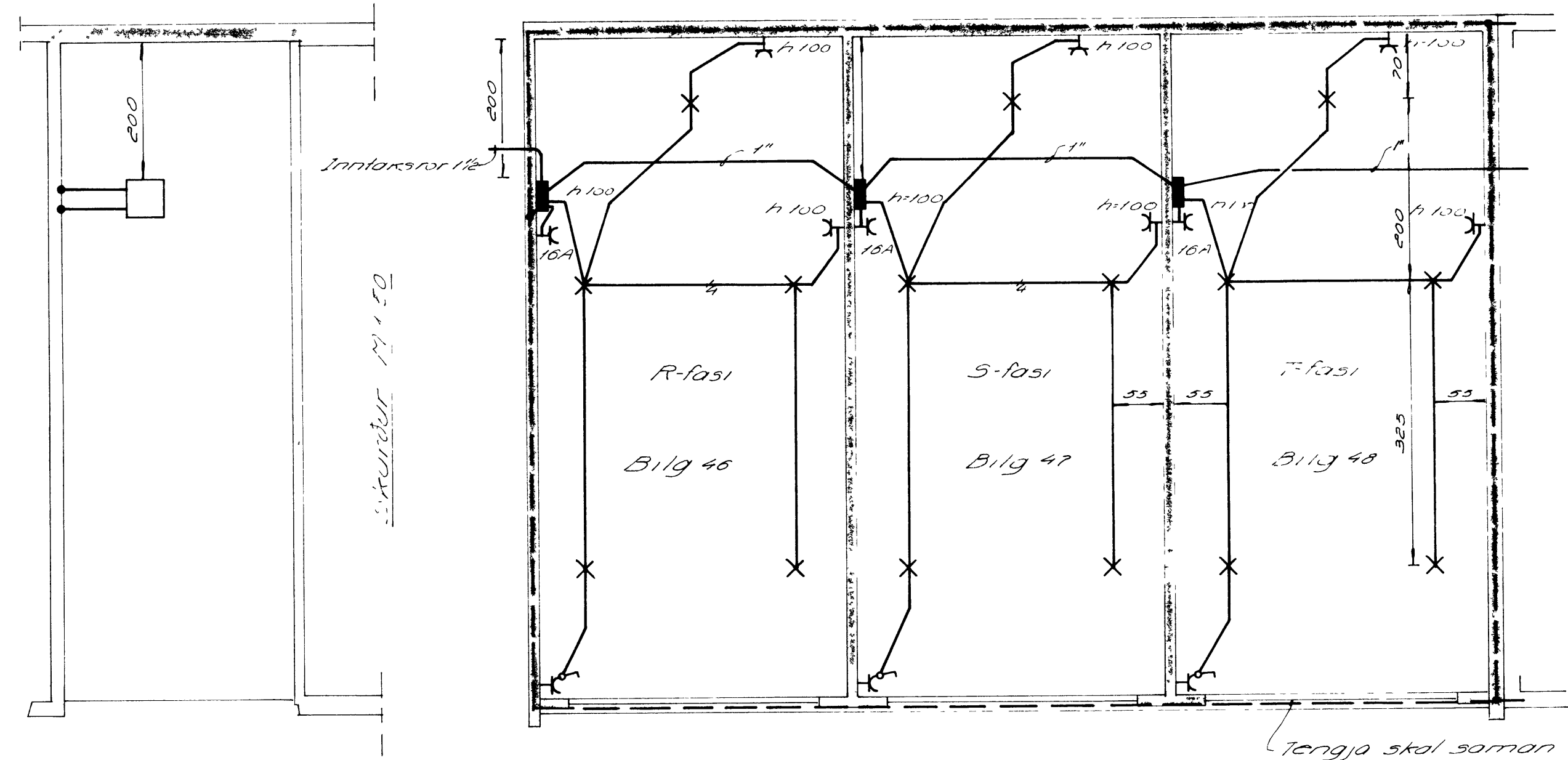
Grunnmynd nr 1.5 Tengja skal samant og neðstu jarnin í sokkulinum
