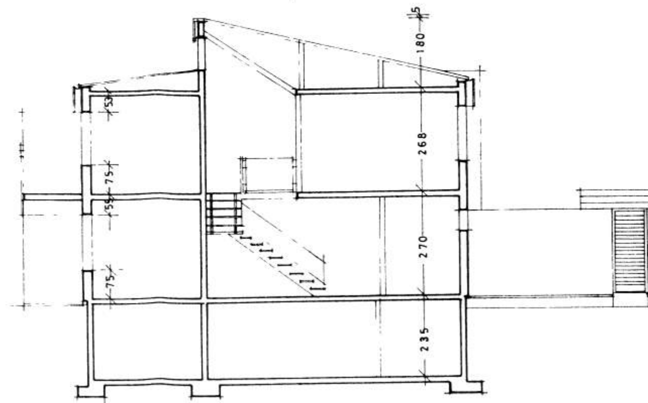
SNIÐ
