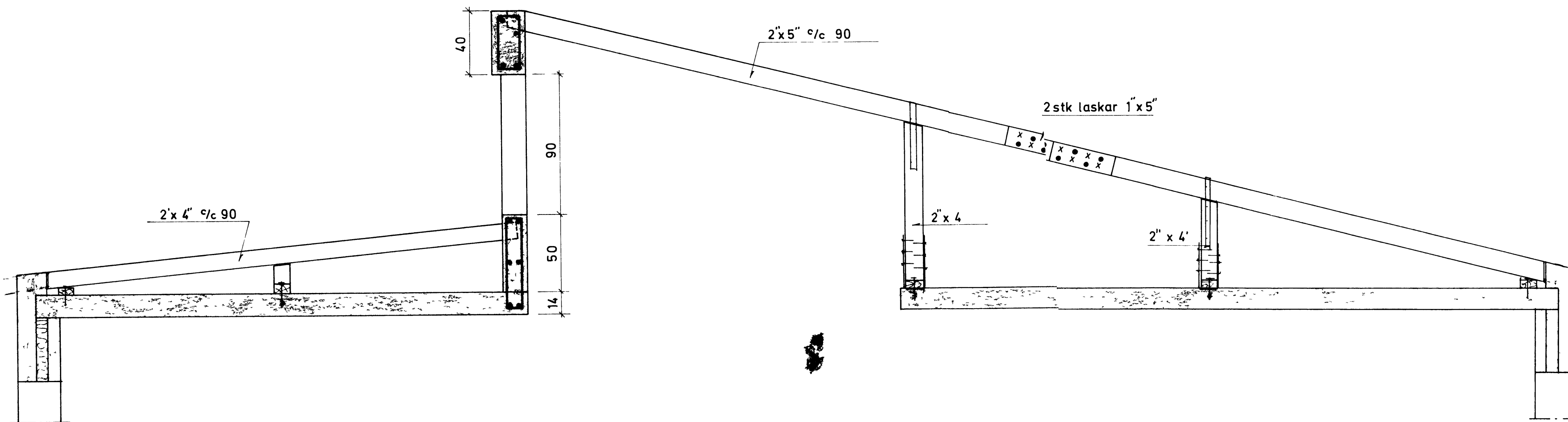
SNIÐ A-A, 1:20
