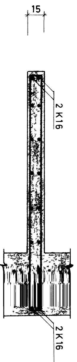
A - A, 1 20
