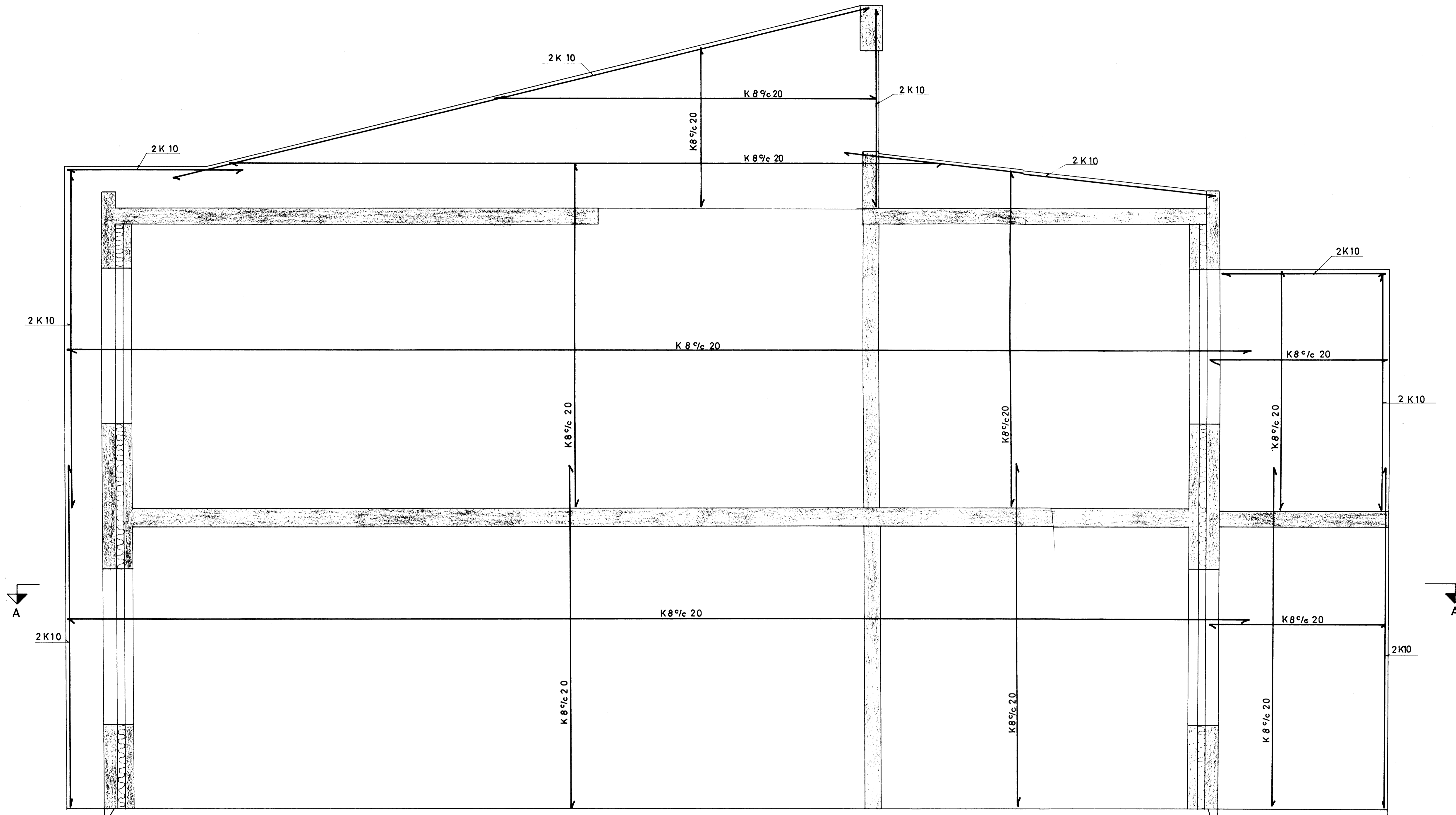
SNID A-A 1:20
