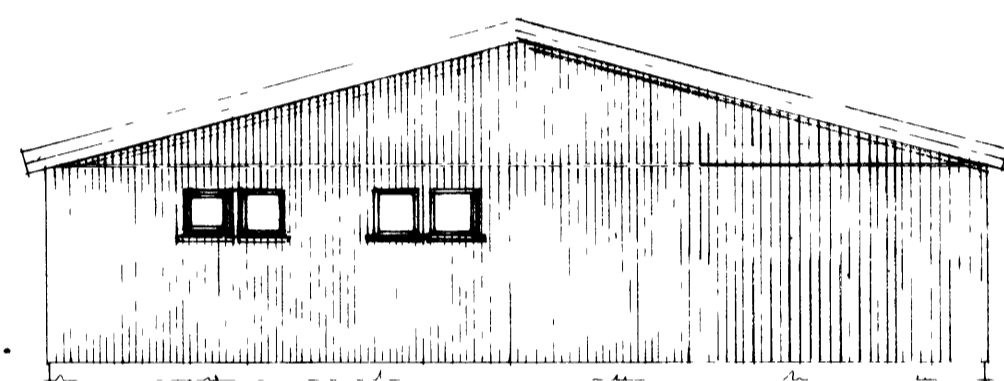
SUÐURHLÍÐ
