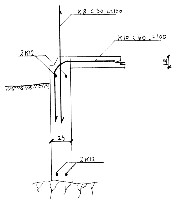
SNID A-A MKv. 1:20
