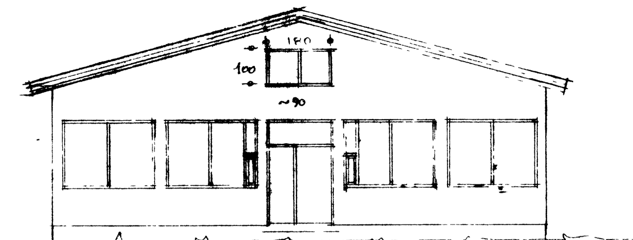
NORÐUR HLIÐ 1:100
