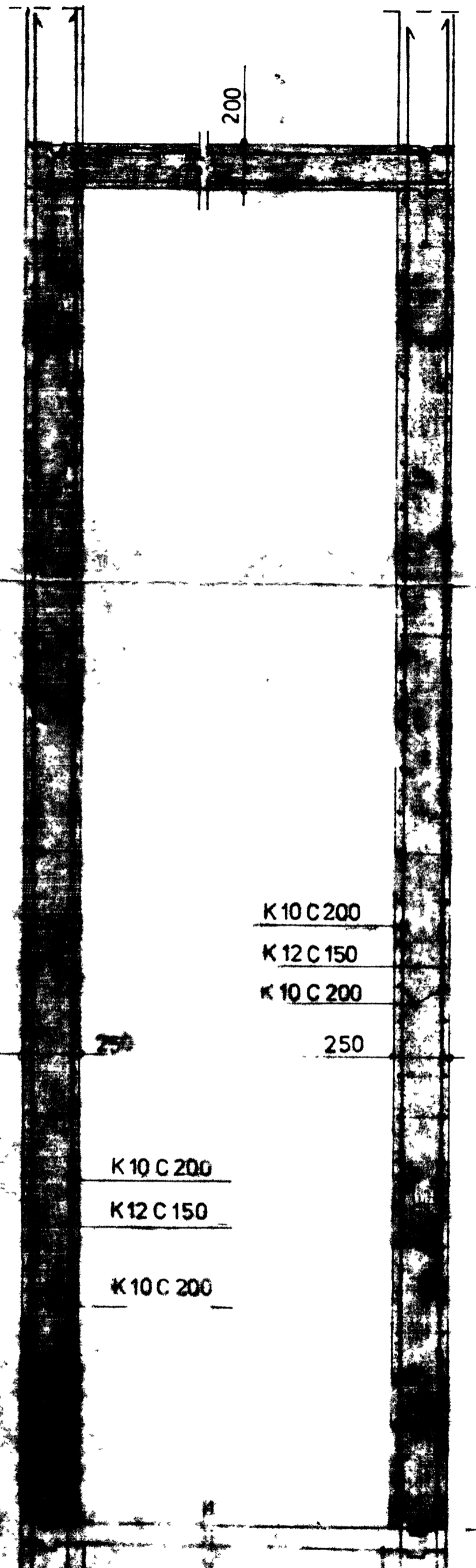
VESTURGAFL AUSTURGAFL SNIÐ I ENDAVEGGI 1:20
