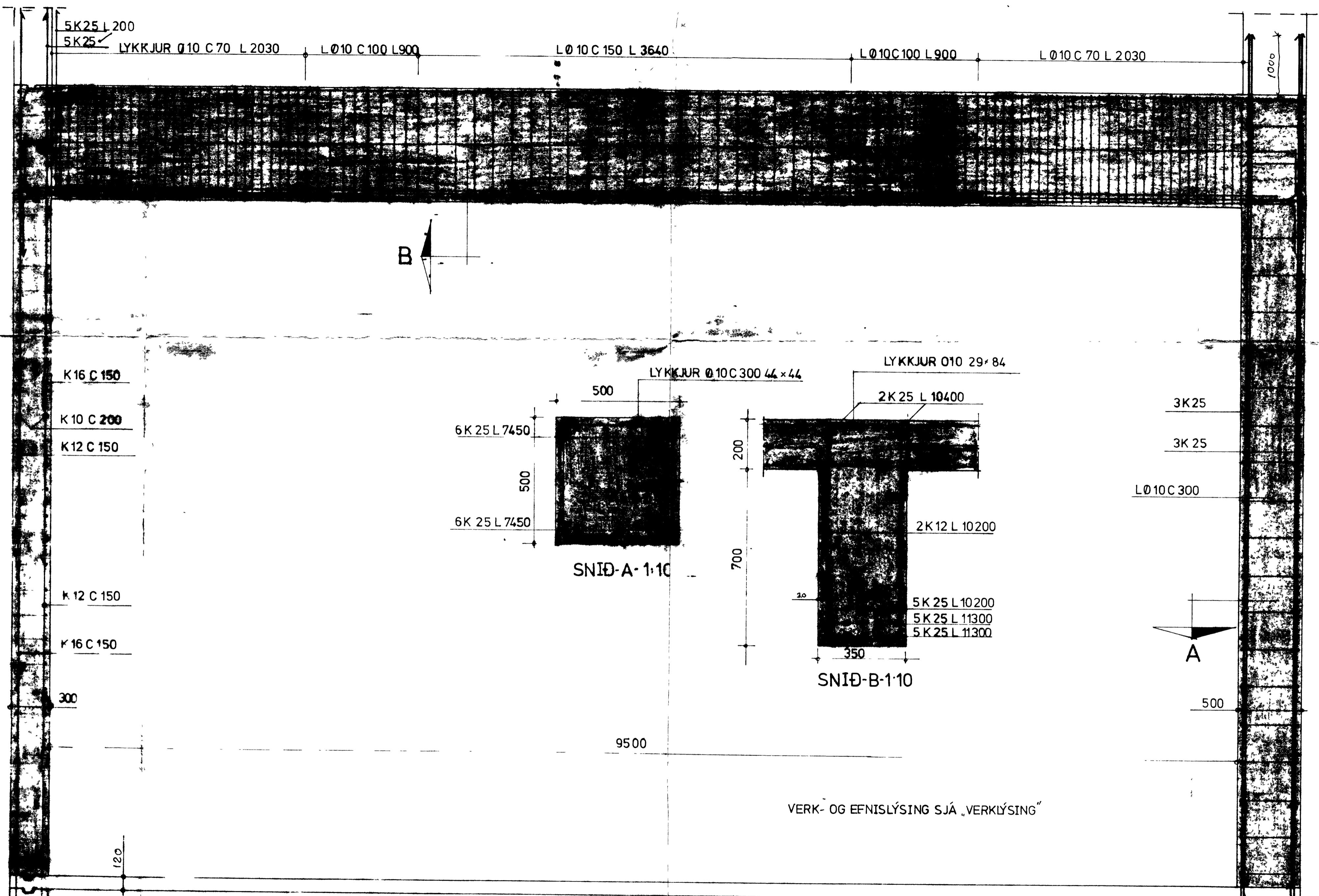
SNIÐ I BITA SÚLUR OG LANGVEGG-1:20
