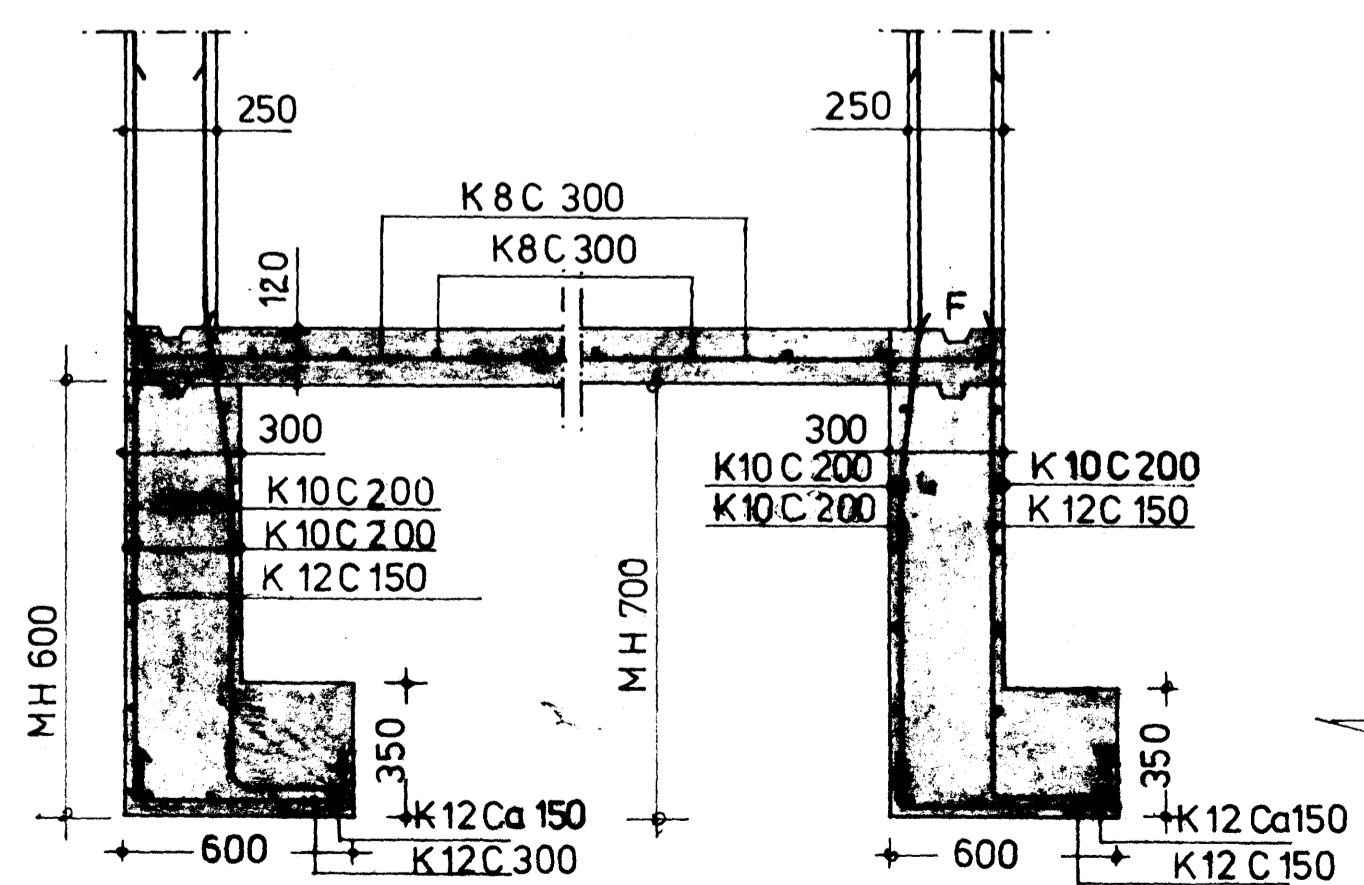
SNID-B-1:20
