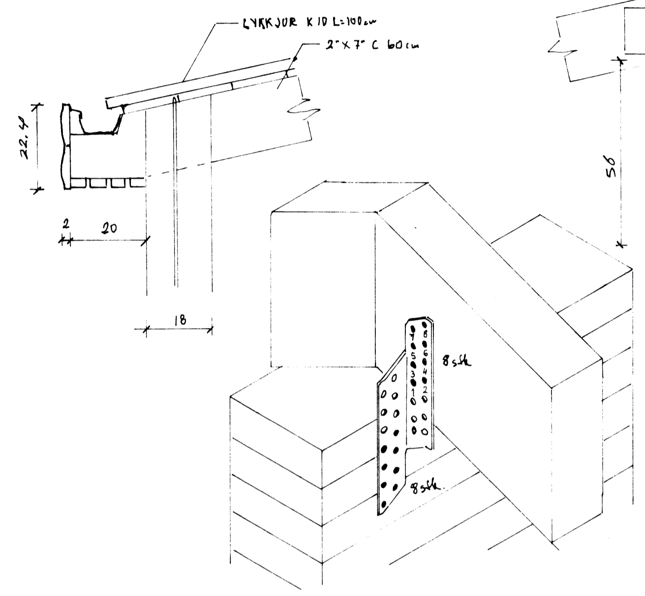
SNID 'I UNDIRSTÖÐU ÖB VEGG MKV 1:10
