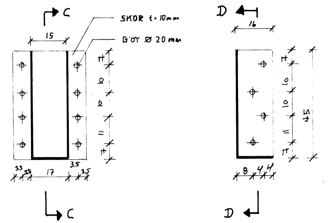
SKOR FYRIR L'IMTRE MKV 1:10
