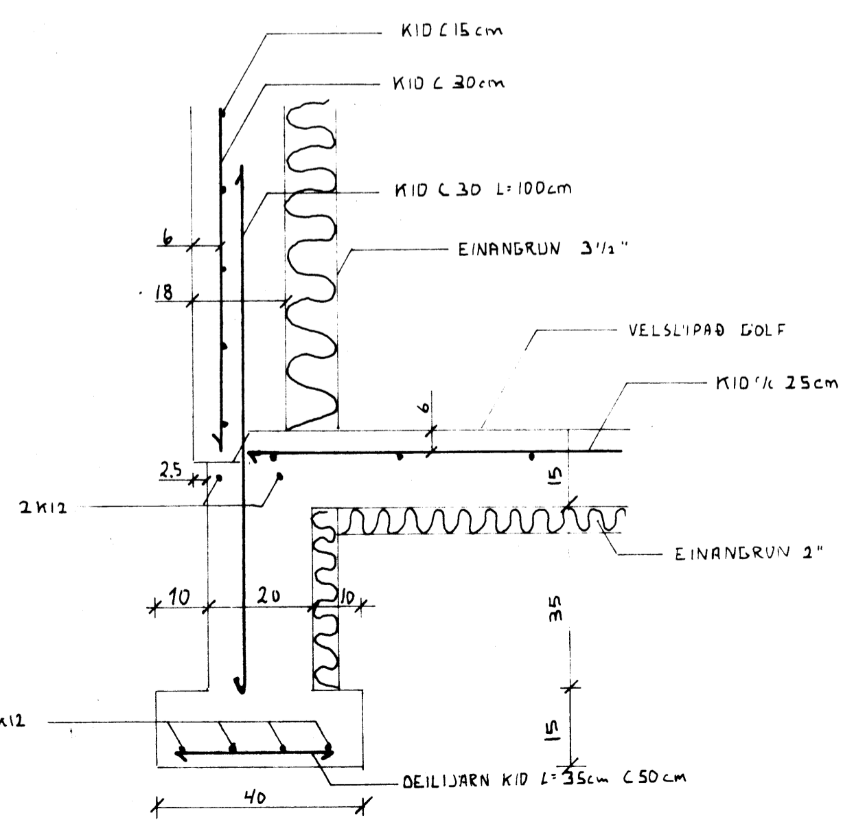
SNID 'I UNDIRSTÖÐU ÖB VEGG MKV 1:10
