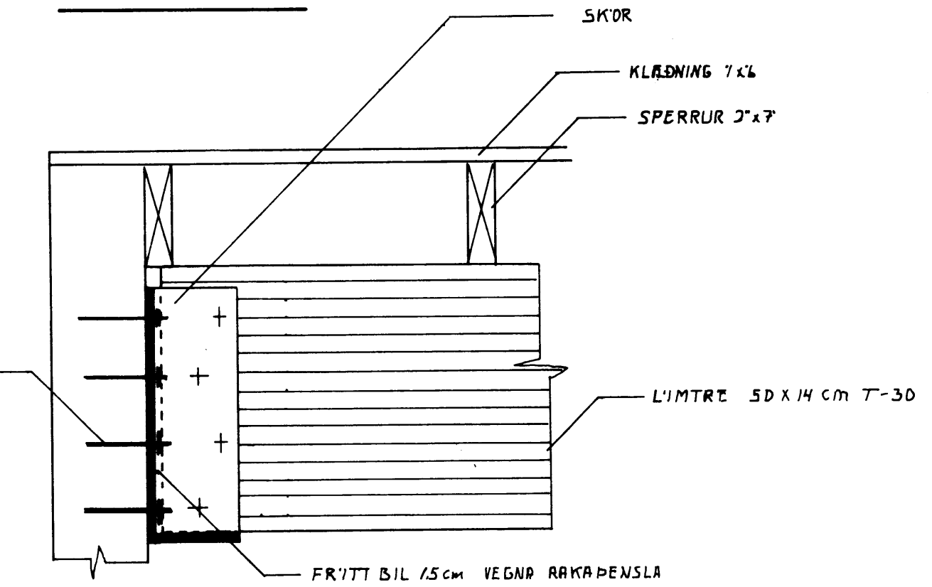
SKOR FYRIR LÍMTRE VÍÐ ÚTVEGG MKV 1:10
