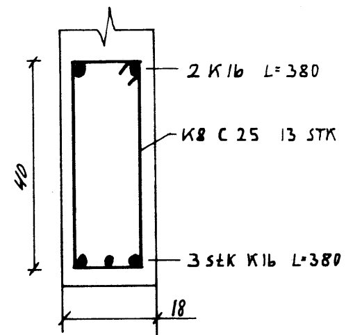
BITI YFIR HURÐ MKV 1:10
