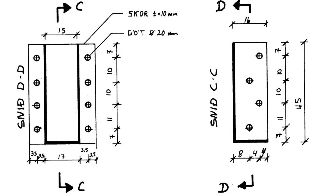
SKOR FYRIR LÍMTRE VÍÐ ÚTVEGG MKV 1:10
