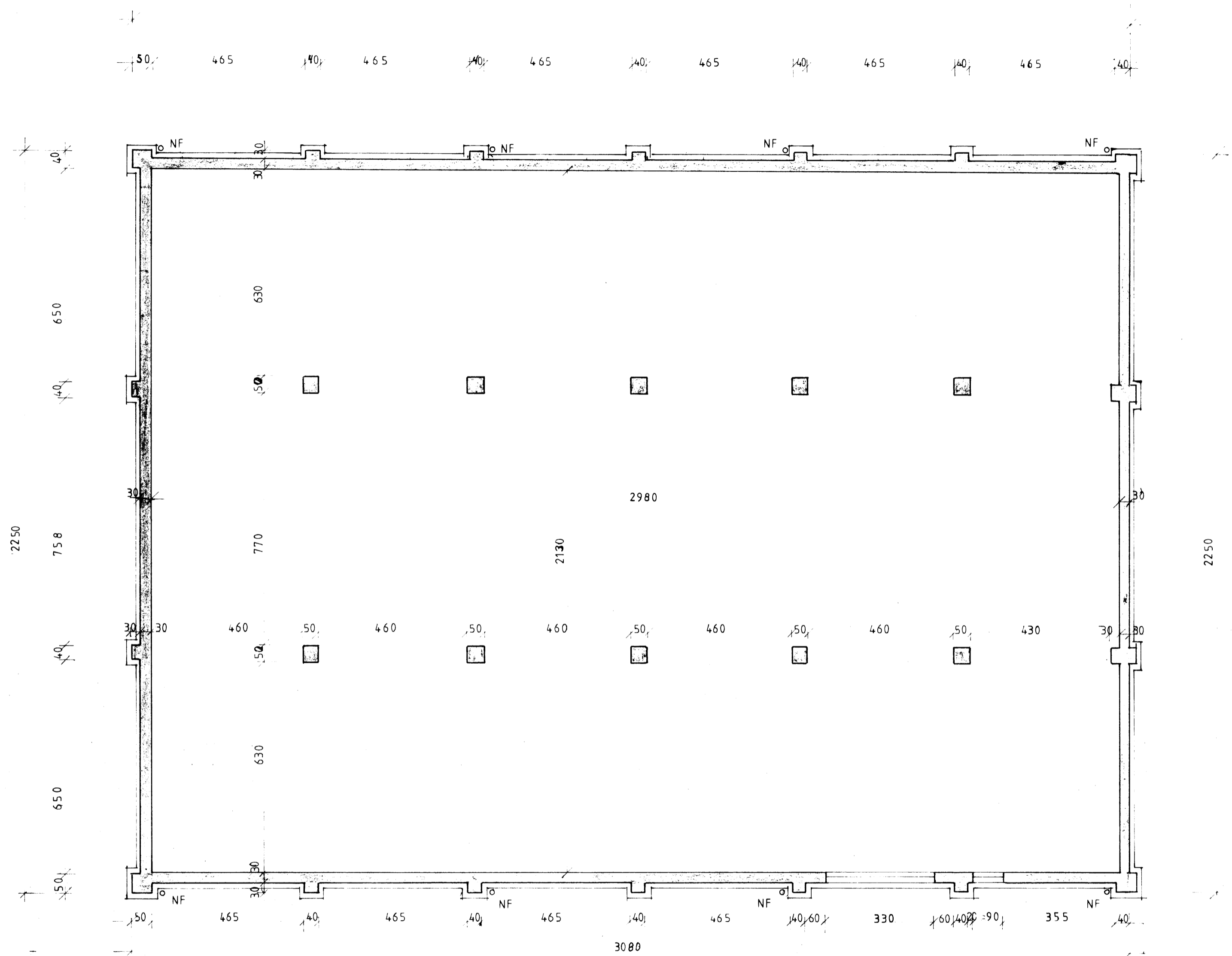
GRUNNMYND 2 HÆÐ 1:100
