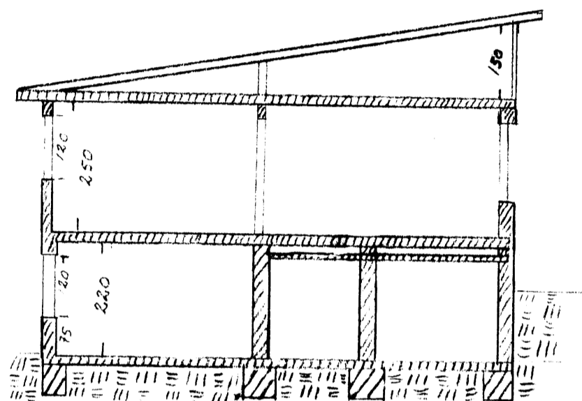
SKURÐUR
