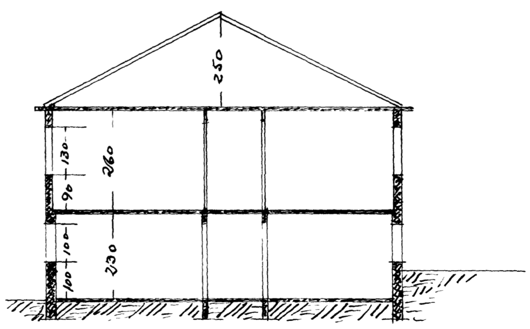
SKURÐUR
