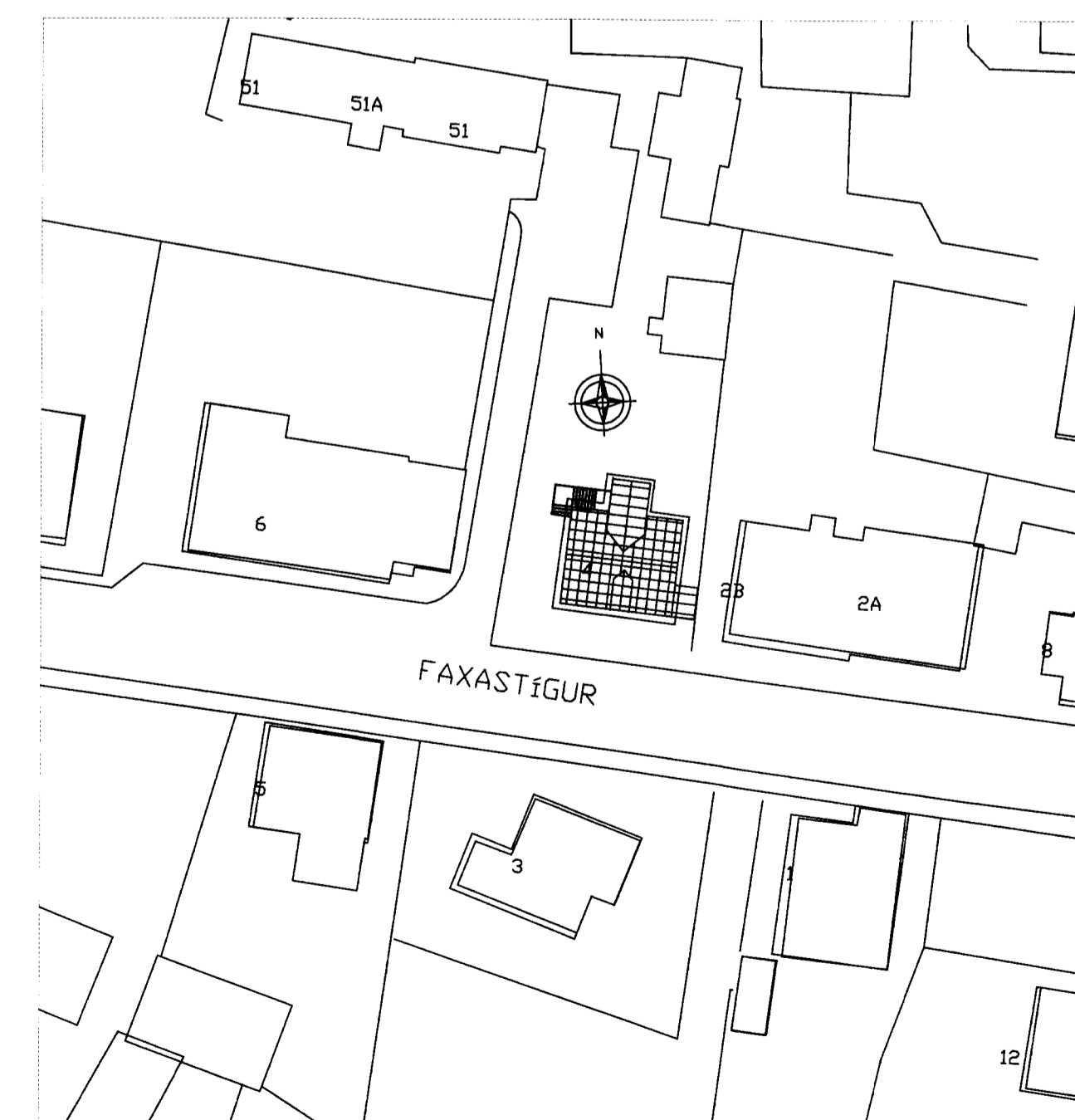
AFSTÖÐUMYND 1:500
