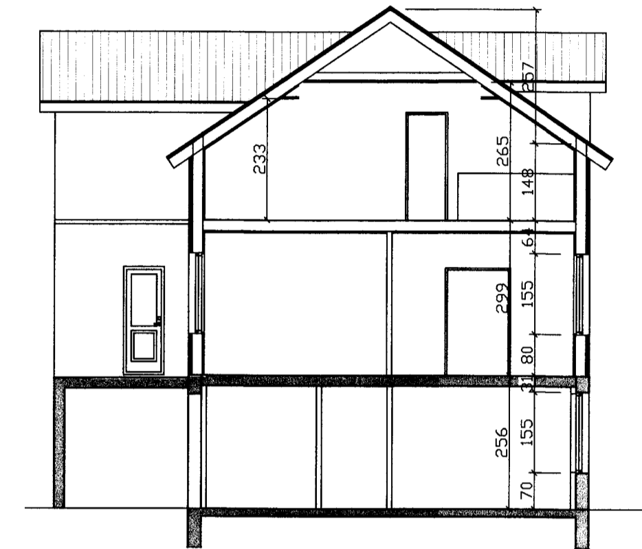
SNID A-A
