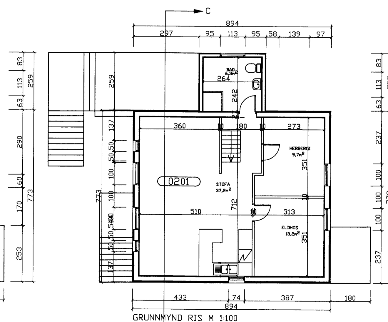
GRUNNMYND RIS M 1:100
