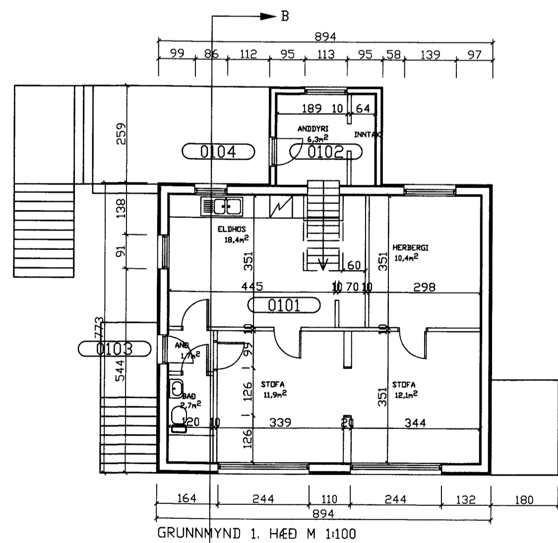
GRUNNMYND 1. HÆÐ M 1:100
