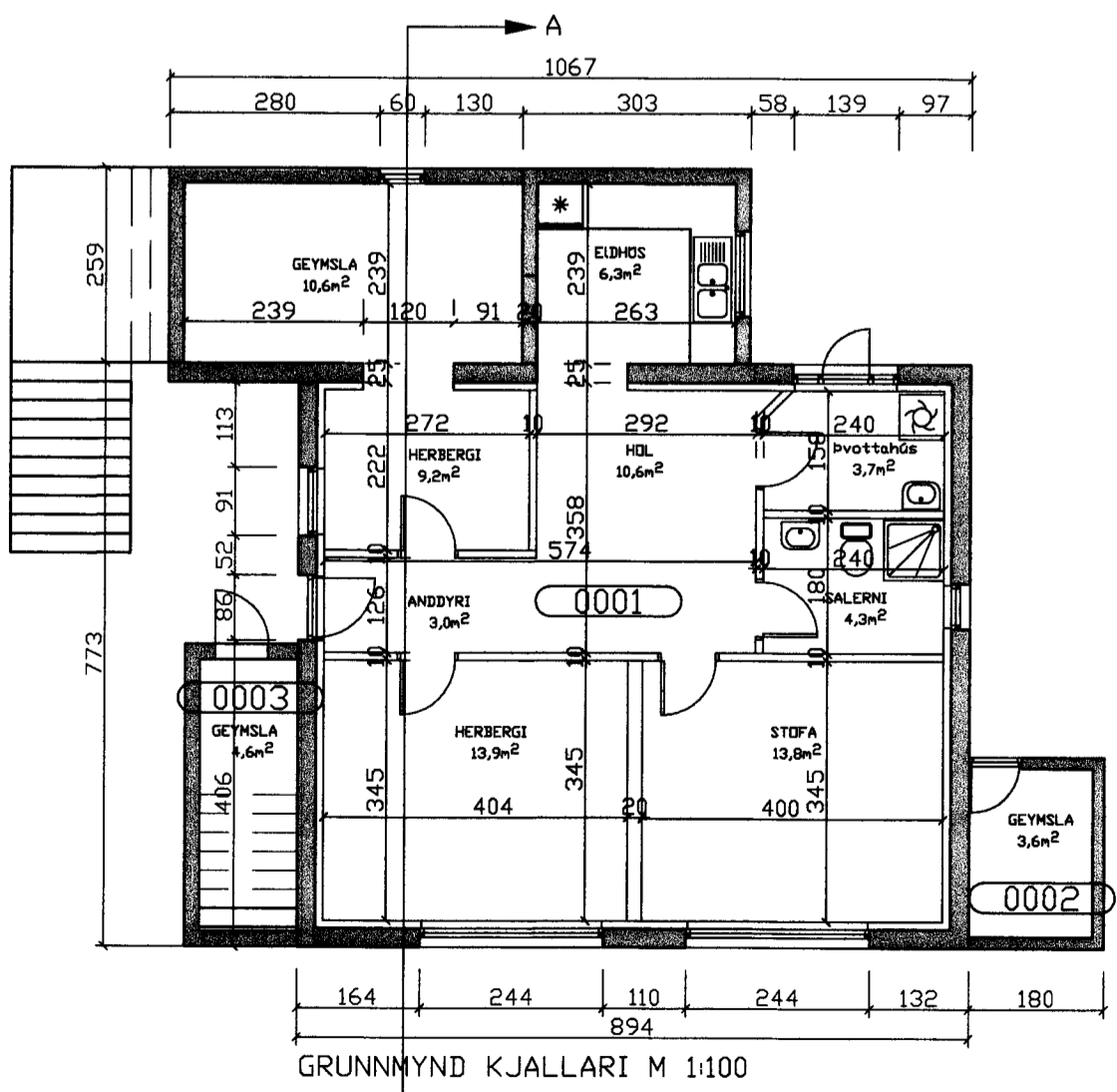
GRUNNMYND KJALLARI M 1:100
