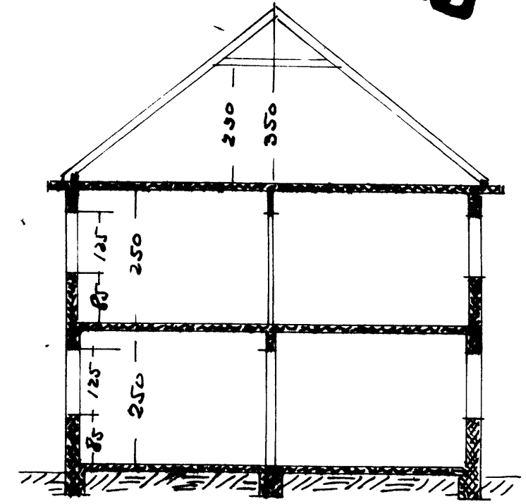
SKURÐUR
