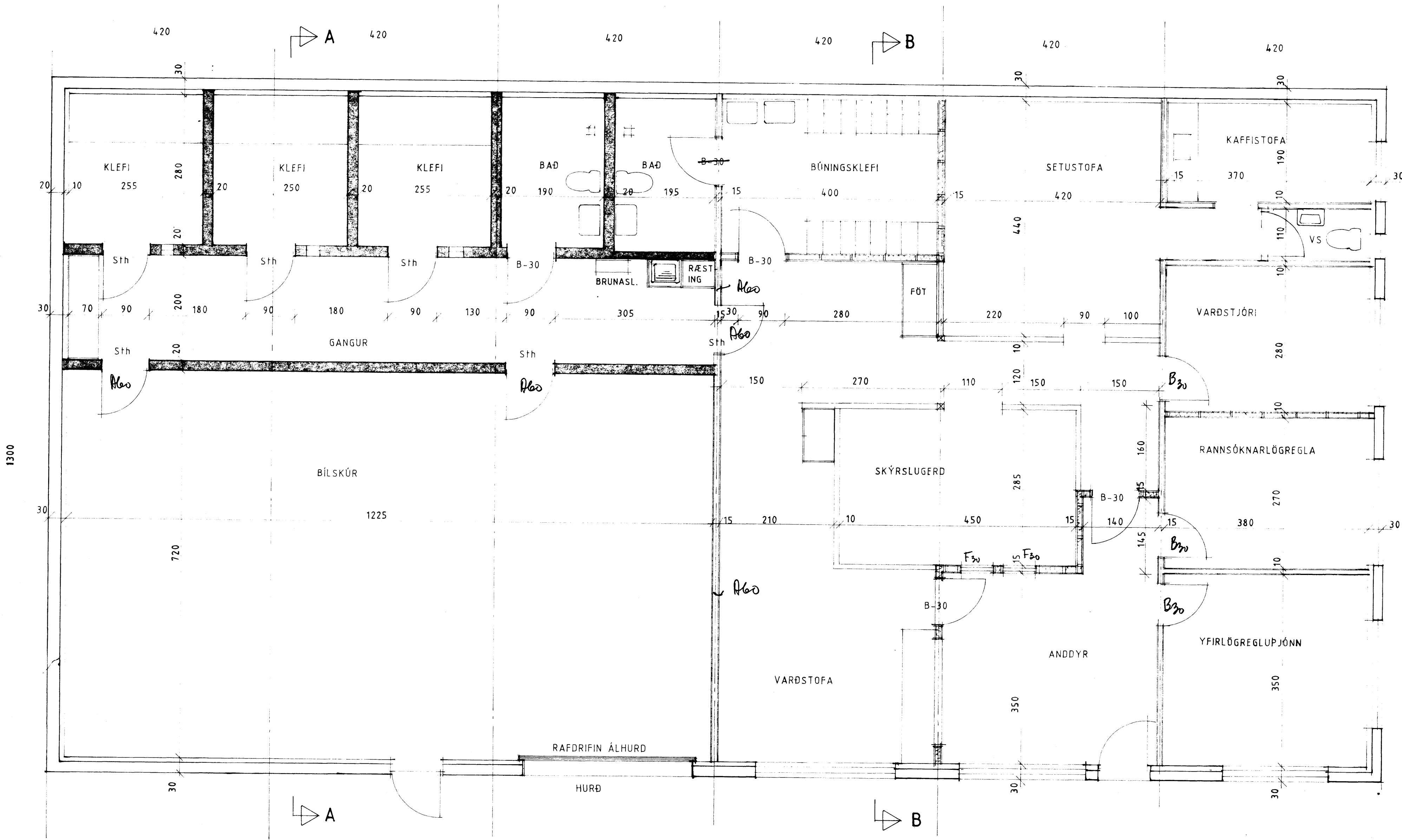
GRUNNMYND Mkv 1:50
