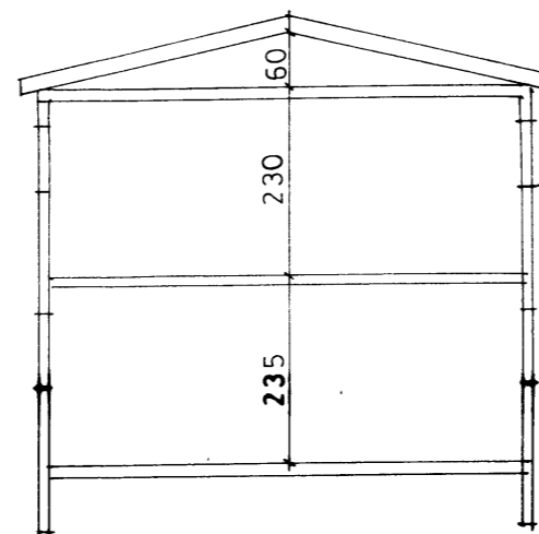
SNIÐ
