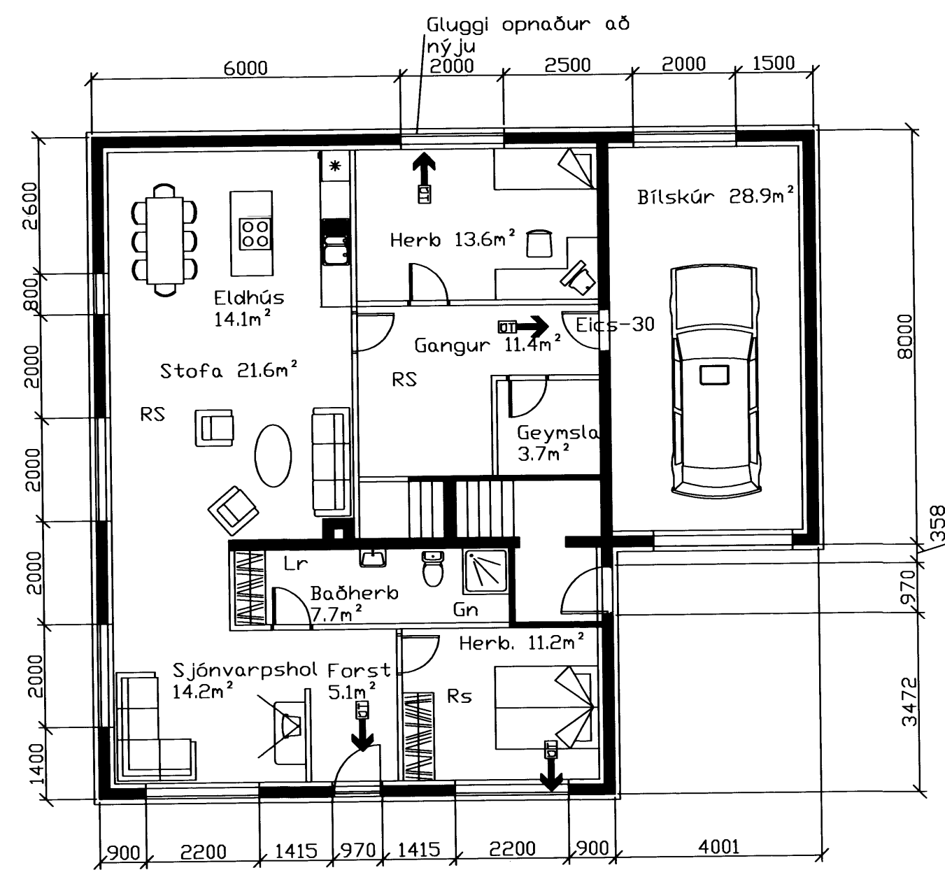
Grunnmynd 1 hæð mkv 1:100
