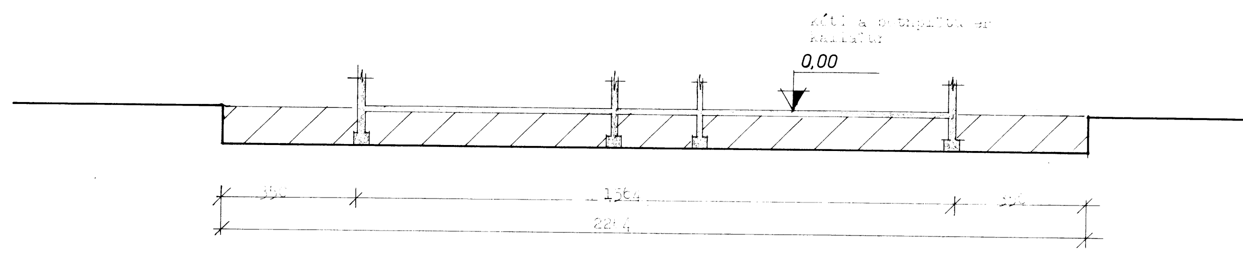
Snid A-A
