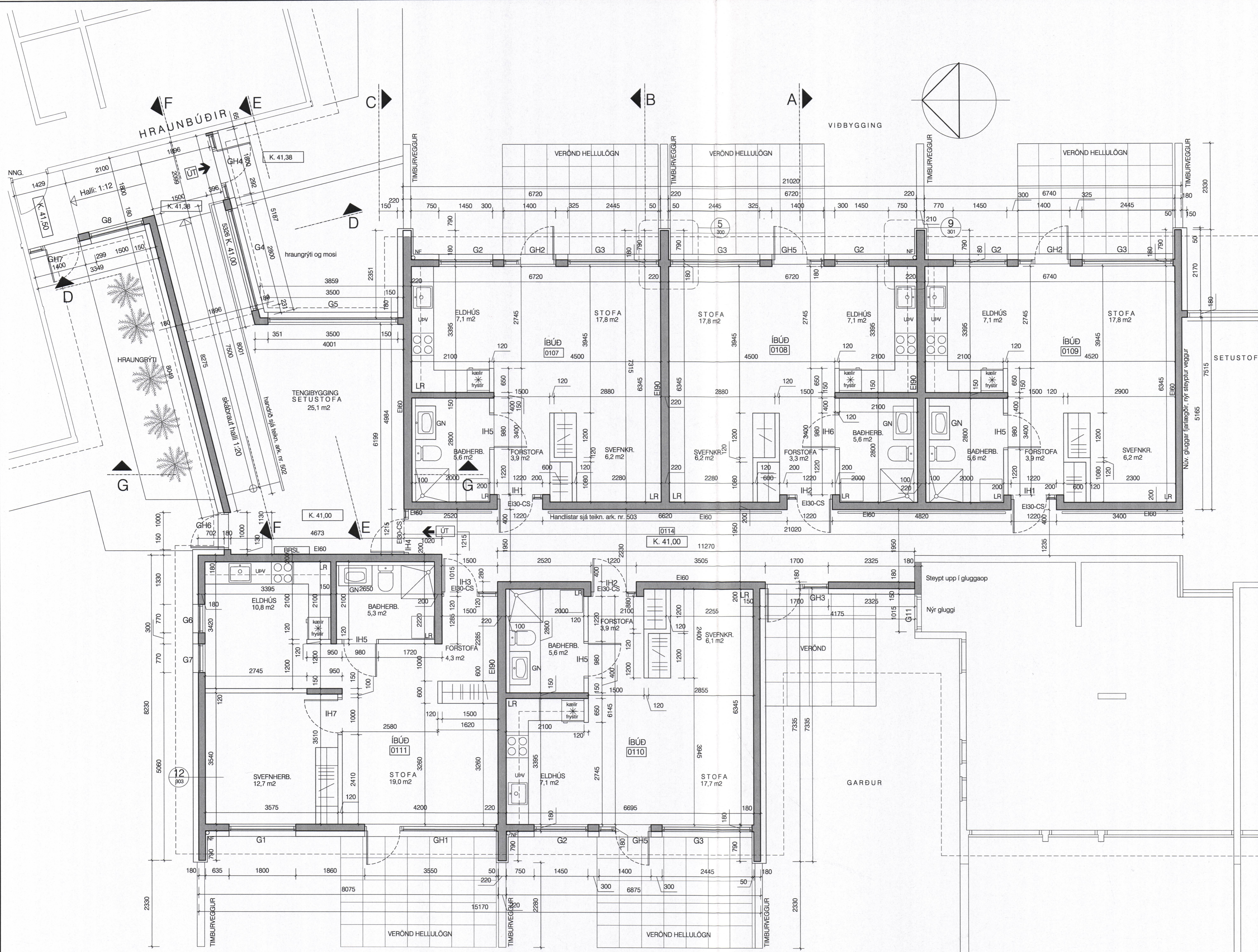
GRUNNMYND 1. HÆÐAR M. 1:50
