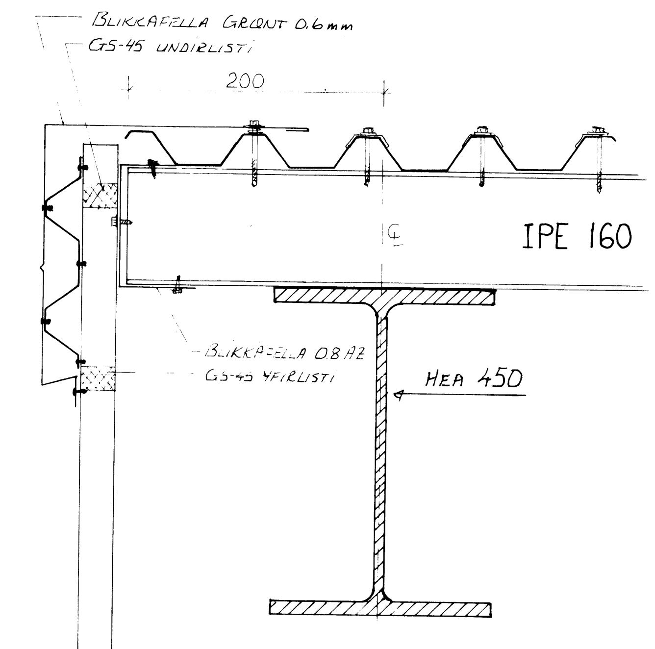
Mynd A-A Mkv. 1:5
