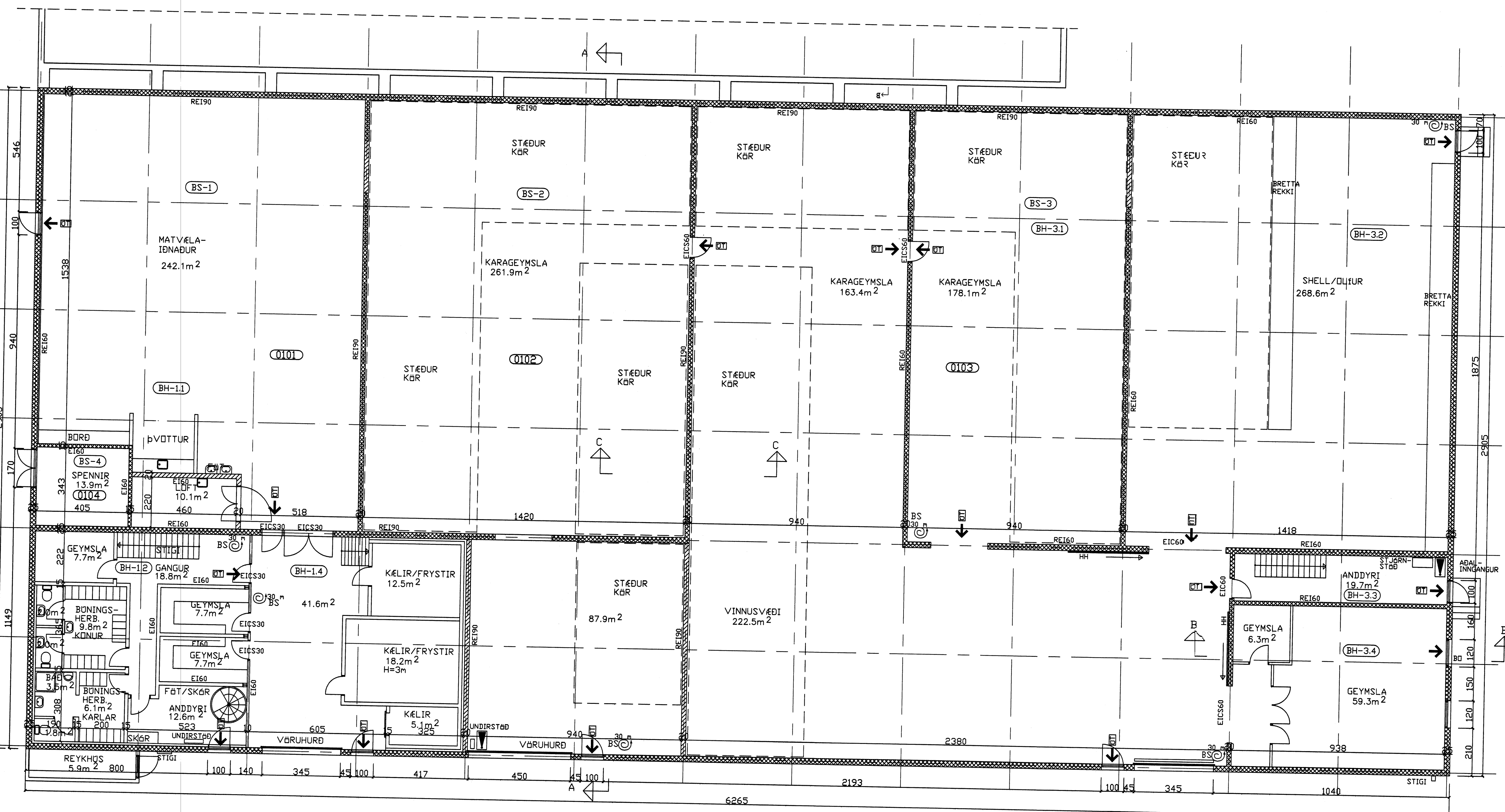
GRUNNMYND 1. HÆÐ
