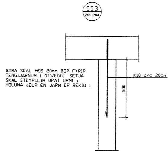
FRAGANGUR OTVEGGJAR VID ELDRÁ HOS M=1:10
