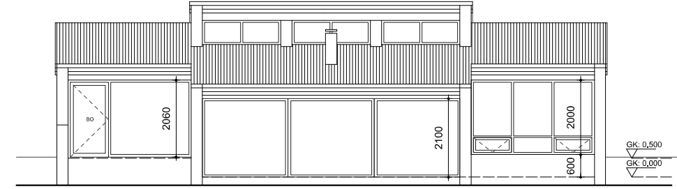
útlit vestur mkv. 1:100
