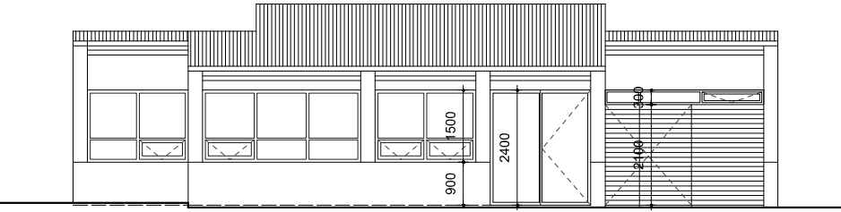
útlit austur mkv. 1:100
