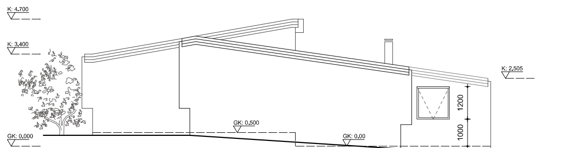
útlit norður mkv. 1:100
