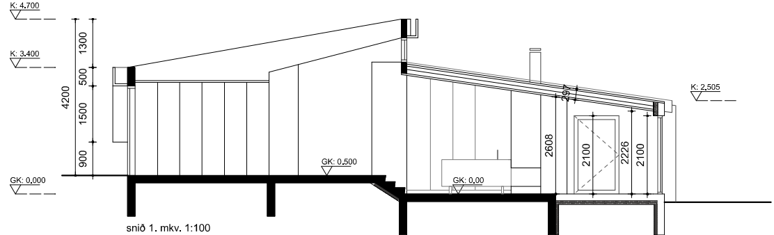
snið 1. mkv. 1:100
