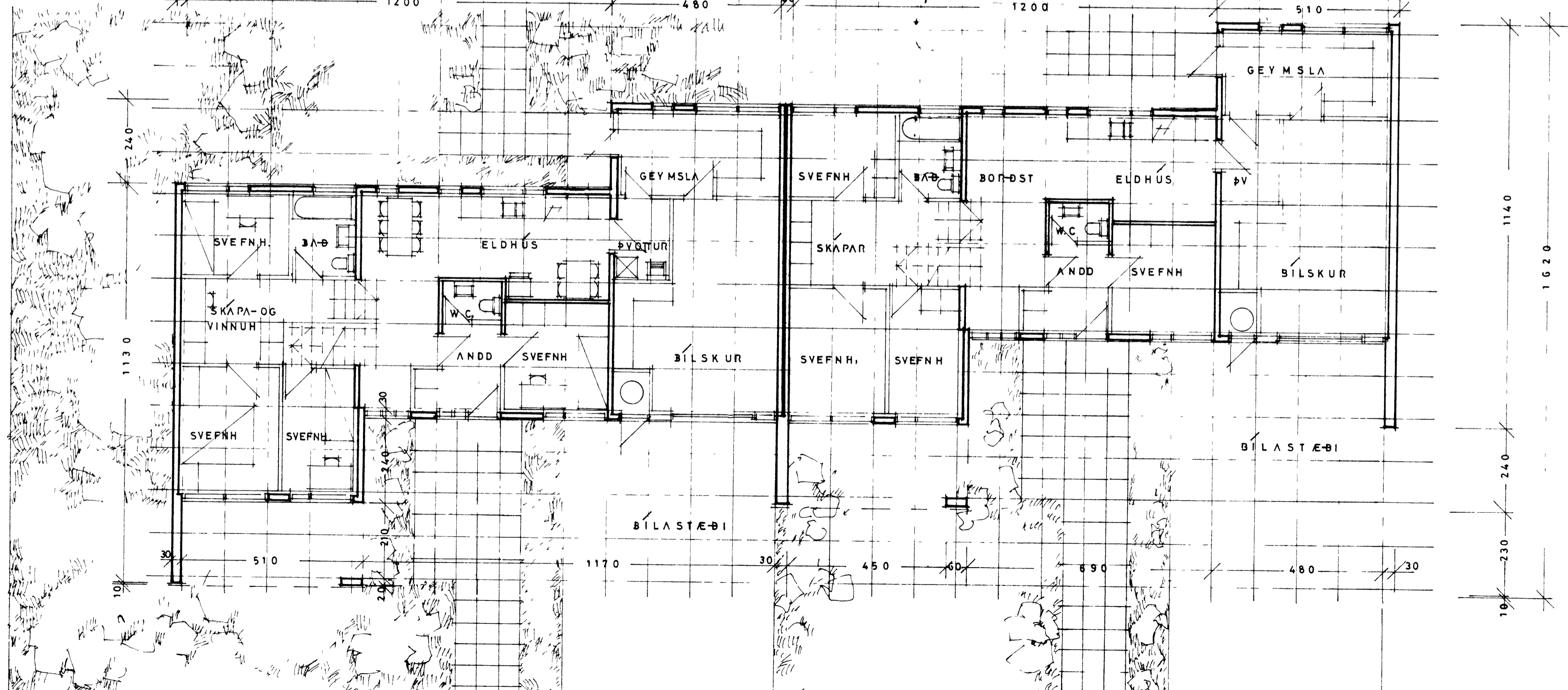
NEÐRI HÆÐ
