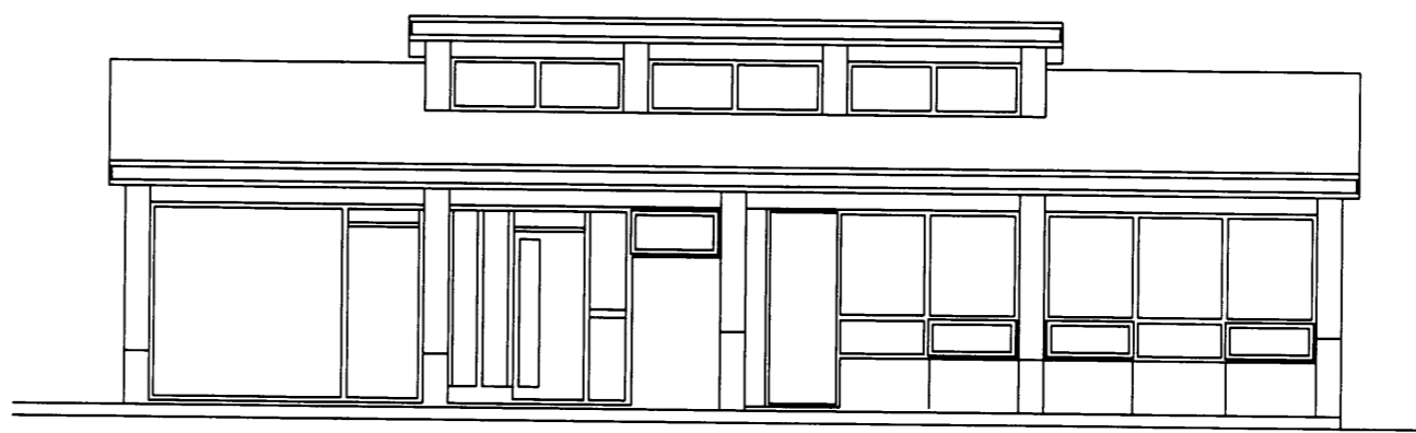
VESTURGAFL
