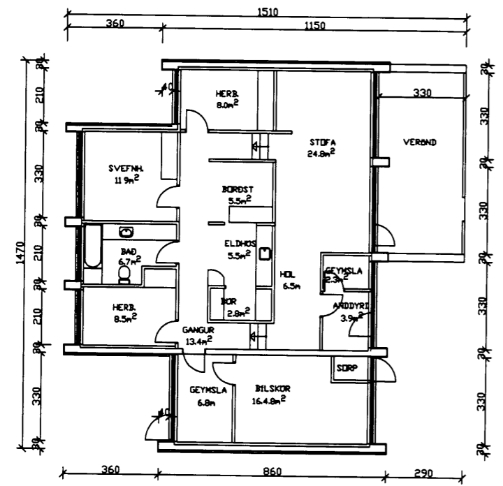
GRUNNMYND 1:50
