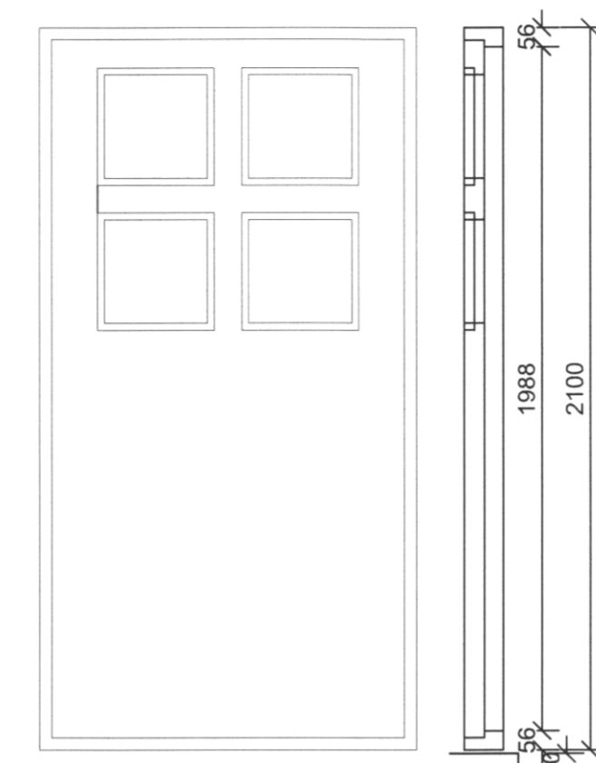
ÚTIHURÐ 1 STK.
