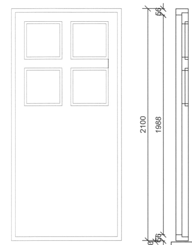
ÚTIHURÐ 1 STK.
