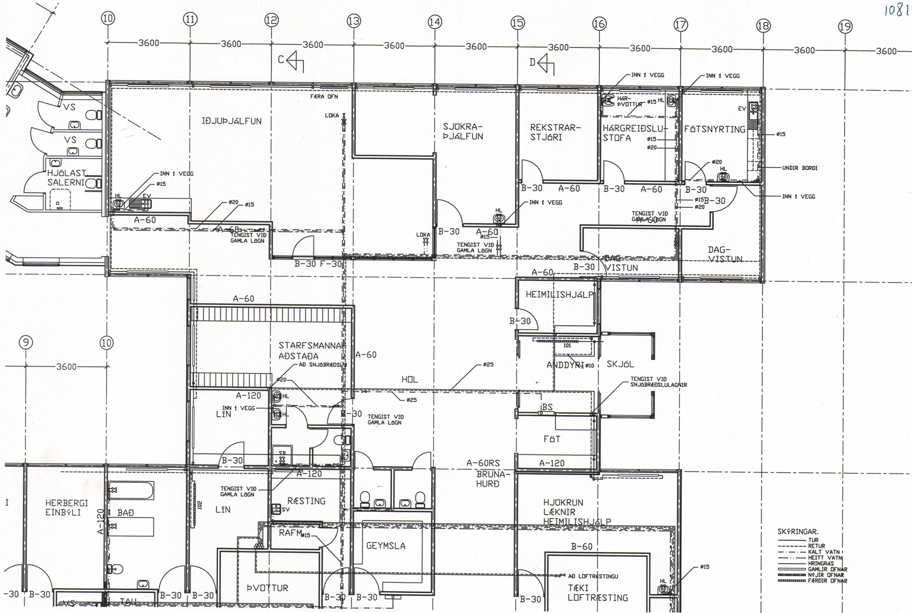
GRUNNMYND NÖRÐURHLUTI M=1:50
