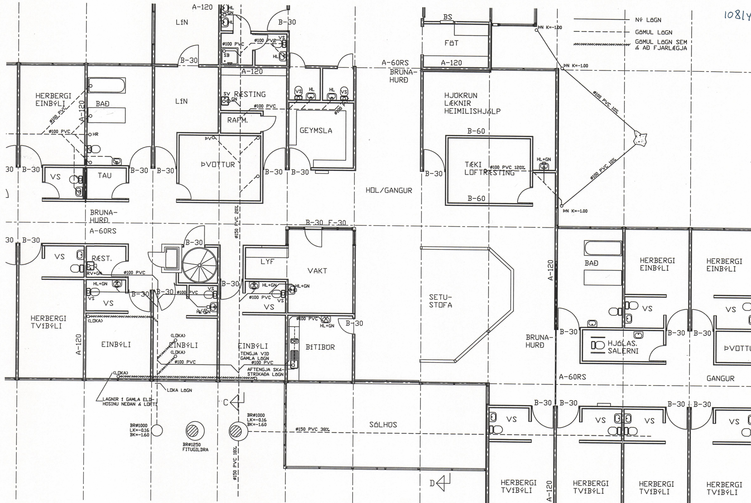
GRUNNMYND SUÐURHLUTI M=1:50
