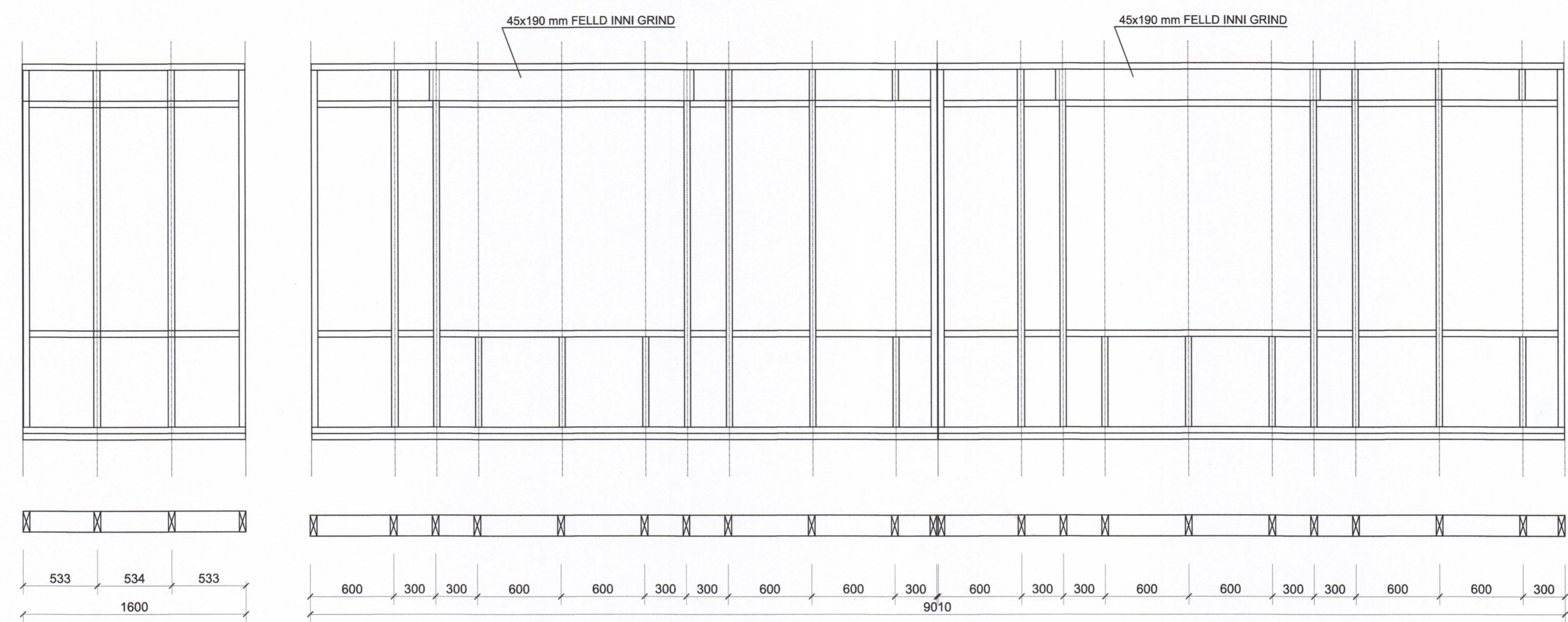
GRIND ÚTVEGGJAR NORÐURHLIÐ
