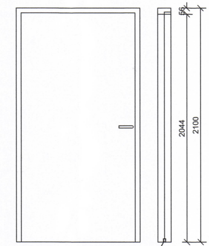
INNIHURÐ H-5 4 STK. M=1:20
