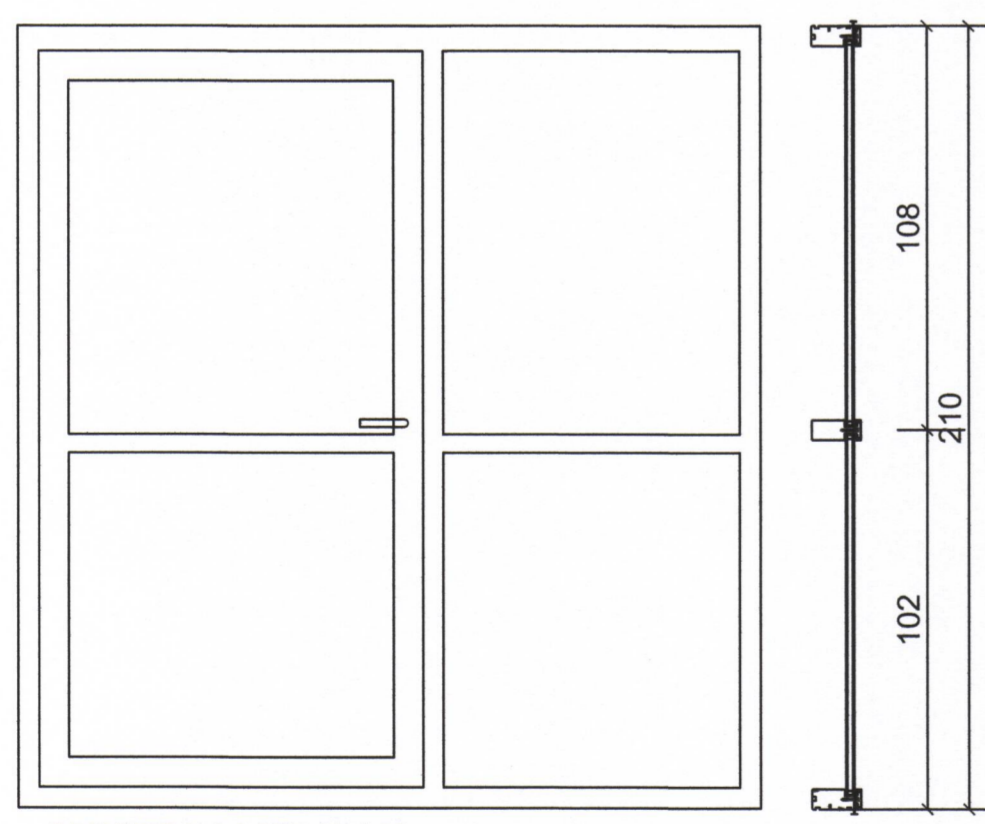
INNIHURÐ H-3 2 STK. M=1:20
