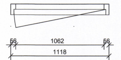
INNIHURÐ H-4 4 STK. M=1:20
