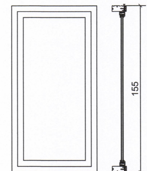
GLUGGI G-3 6 STK. M=1:20
