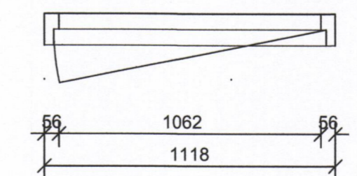
INNIHURÐ H-5 2 STK. M=1:20
