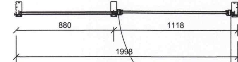
ÚTIHURÐ H-1 1 STK. M=1:20
