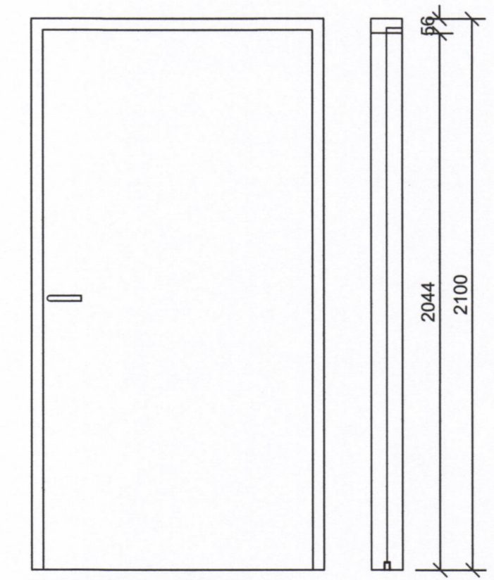
INNIHURÐ H-4 4 STK. M=1:20
