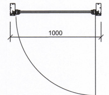
ÚTIHURÐ H-1 1 STK. M=1:20
