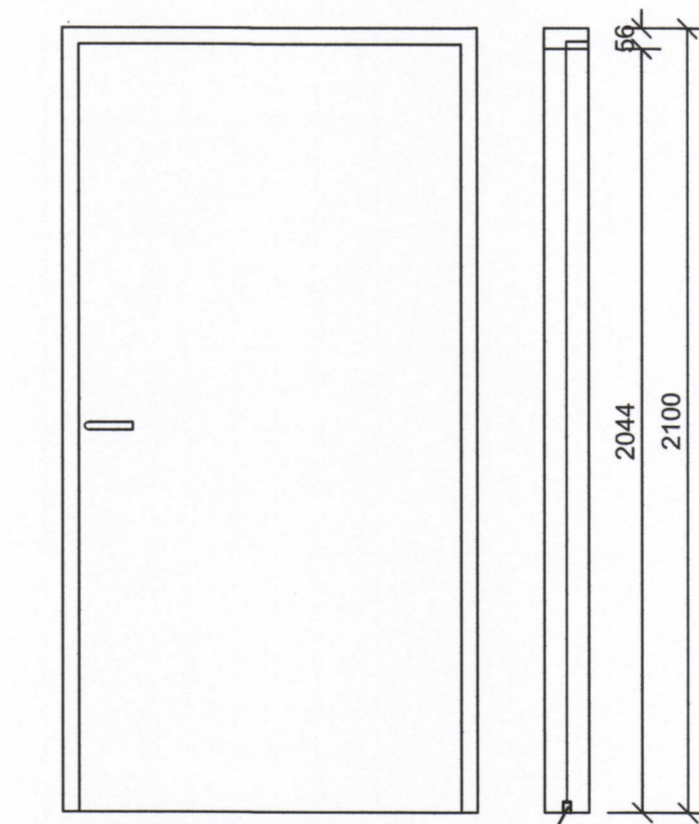
INNIHURÐ H-5 2 STK. M=1:20
