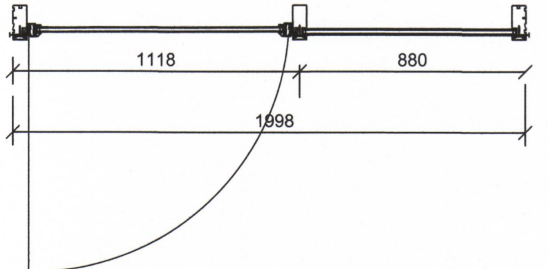
INNIHURÐ H-3 2 STK. M=1:20
