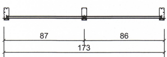
GLUGGI G-1 6 STK. M=1:20
