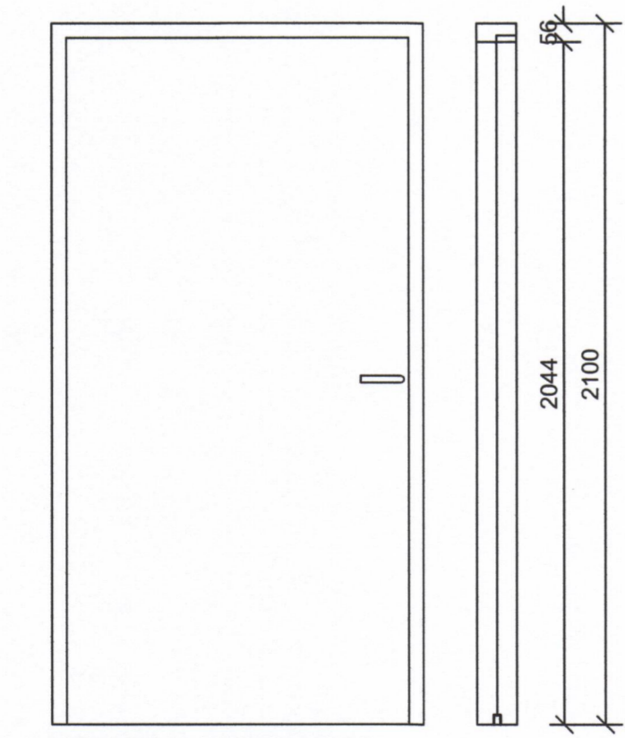
INNIHURÐ H-4 1 STK. M=1:20
