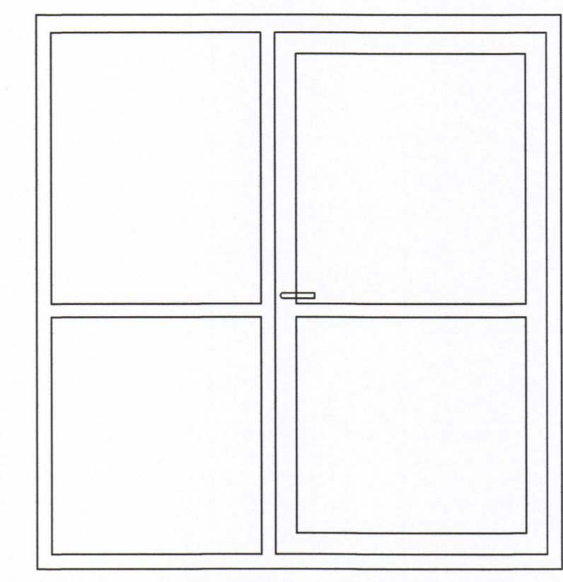
ÚTIHURÐ H-1 1 STK. M=1:20
