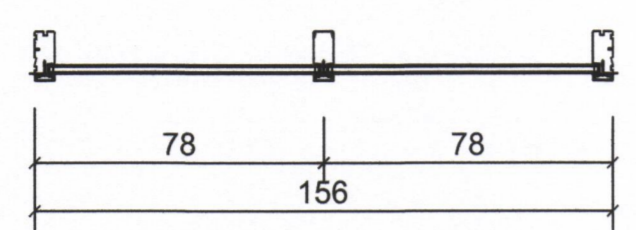
GLUGGI G-2 1 STK. M=1:20
