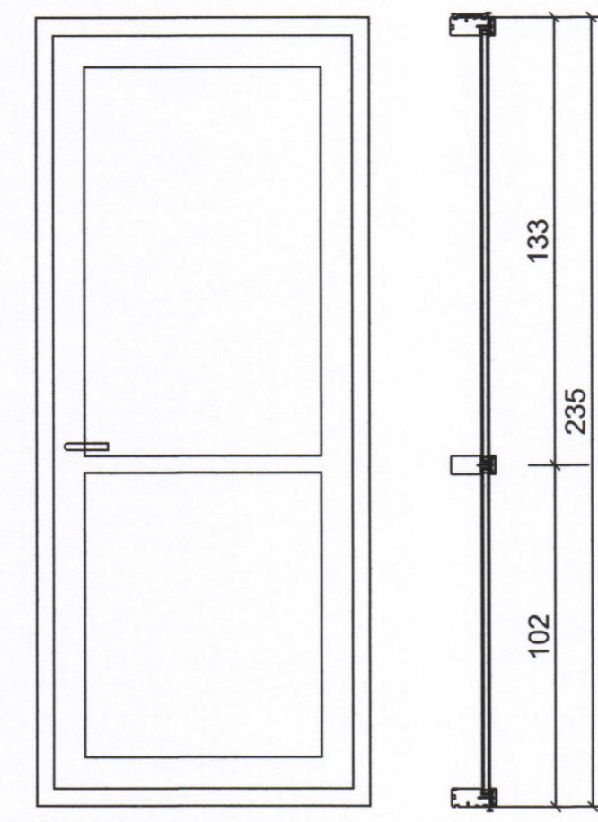
ÚTIHURÐ H-1 1 STK. M=1:20
