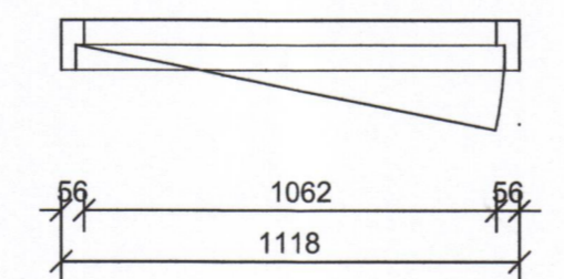
INNIHURÐ H-5 4 STK. M=1:20
