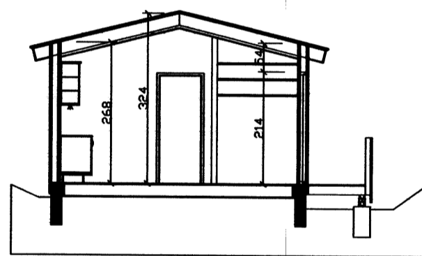
SNID A-A M=1:100
