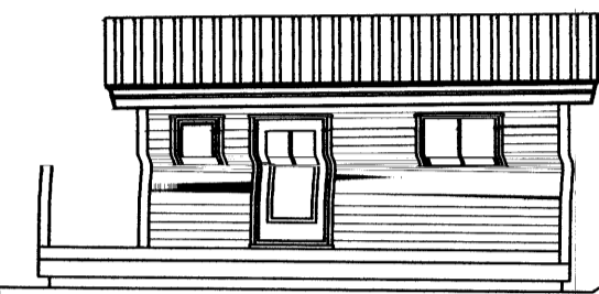
SUB-AUSTUR M=1:100
