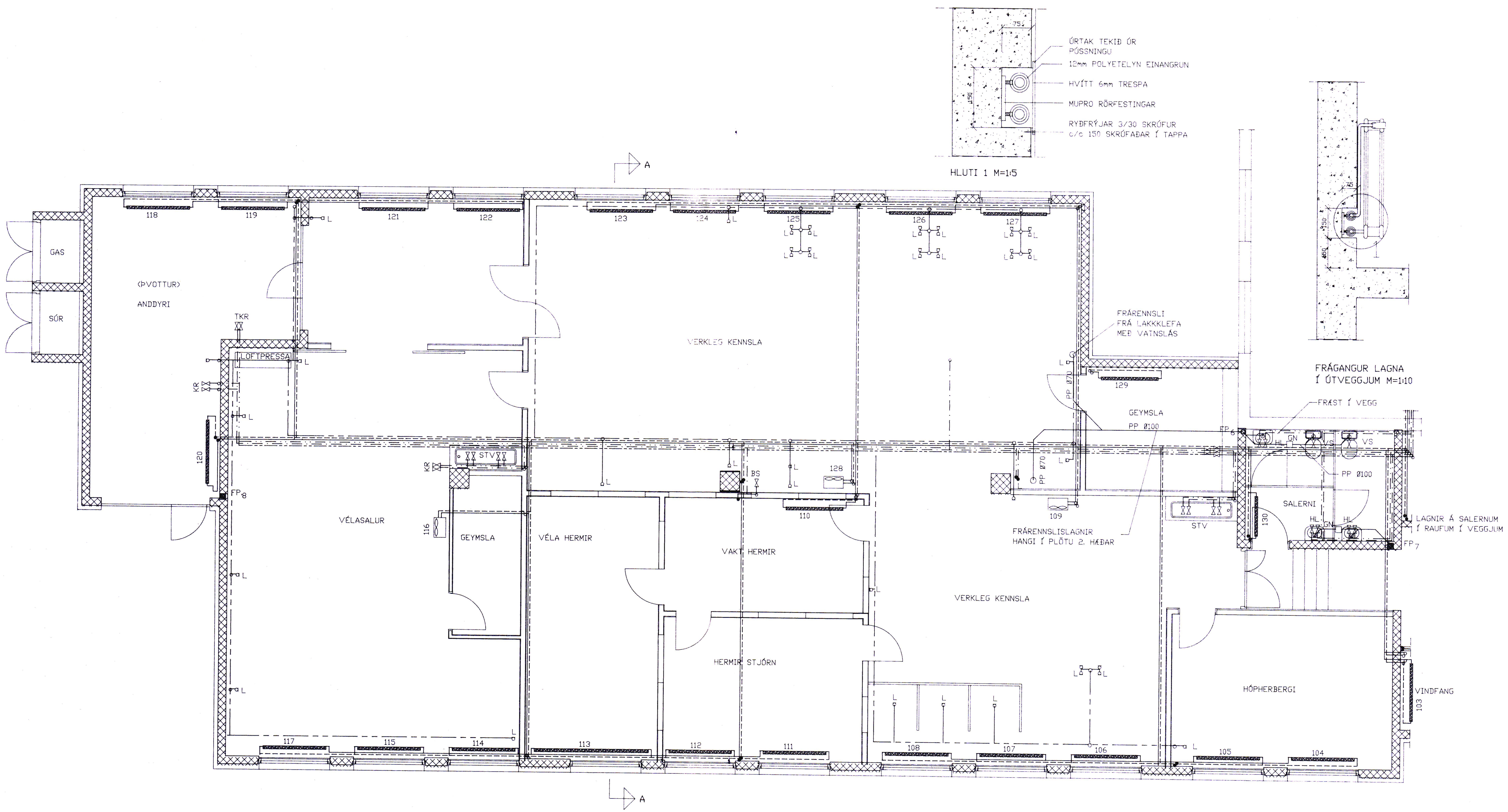
GRUNNMYND 1. HÆÐ M=1:50
