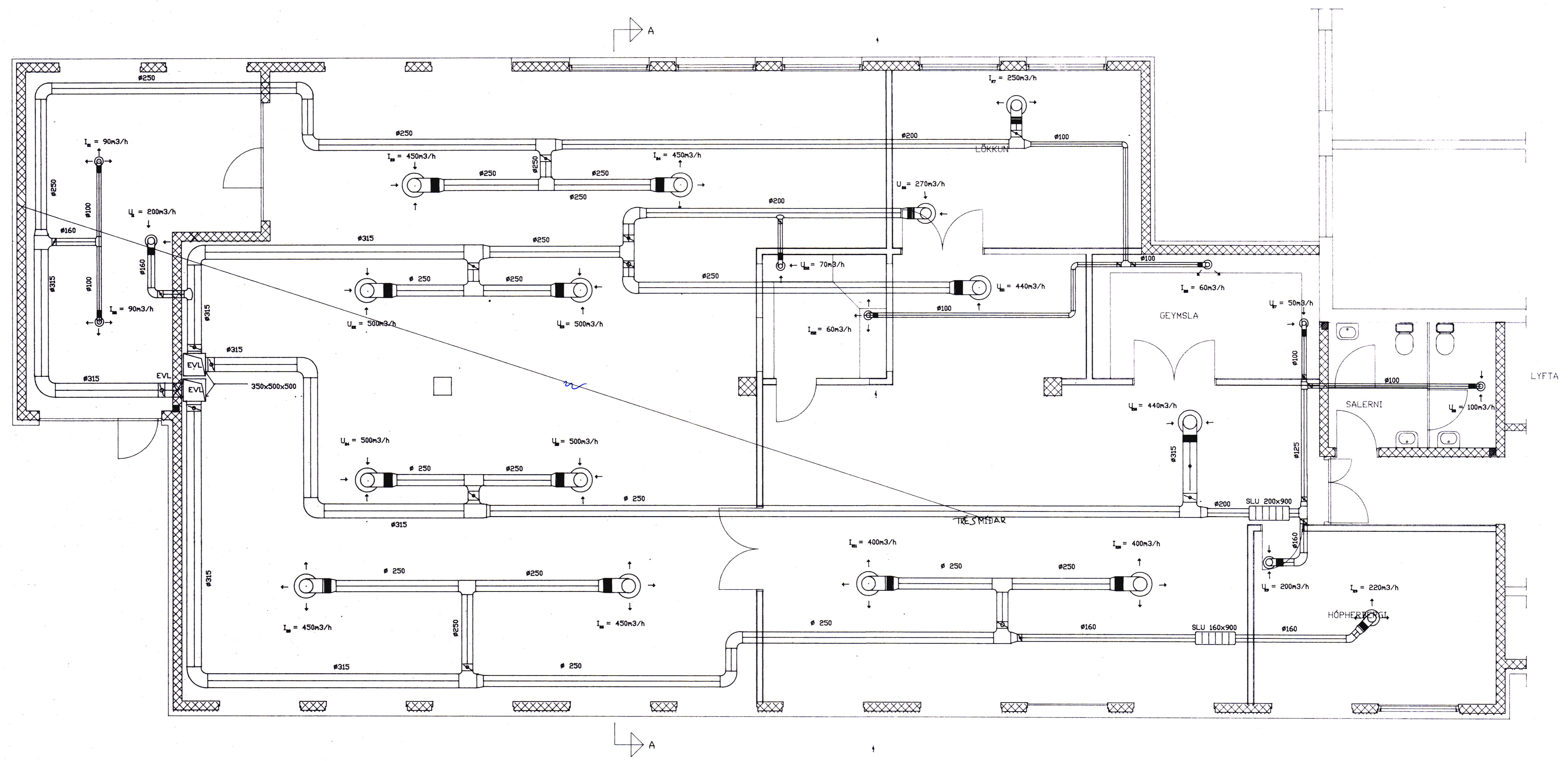
GRUNNMYND 2. HÆÐ M=1:50
