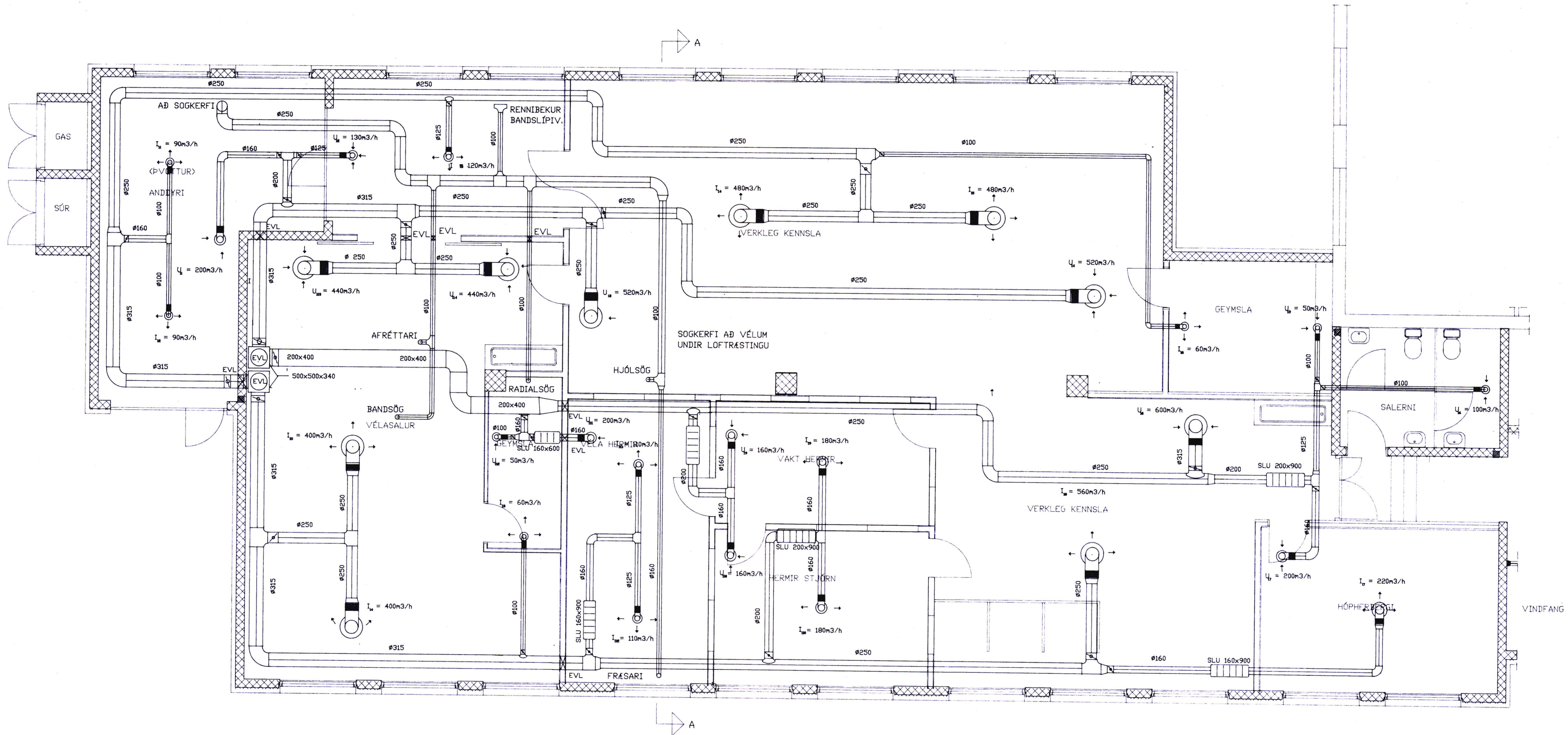
GRUNNMYND 1. HÆÐ M=1:50
