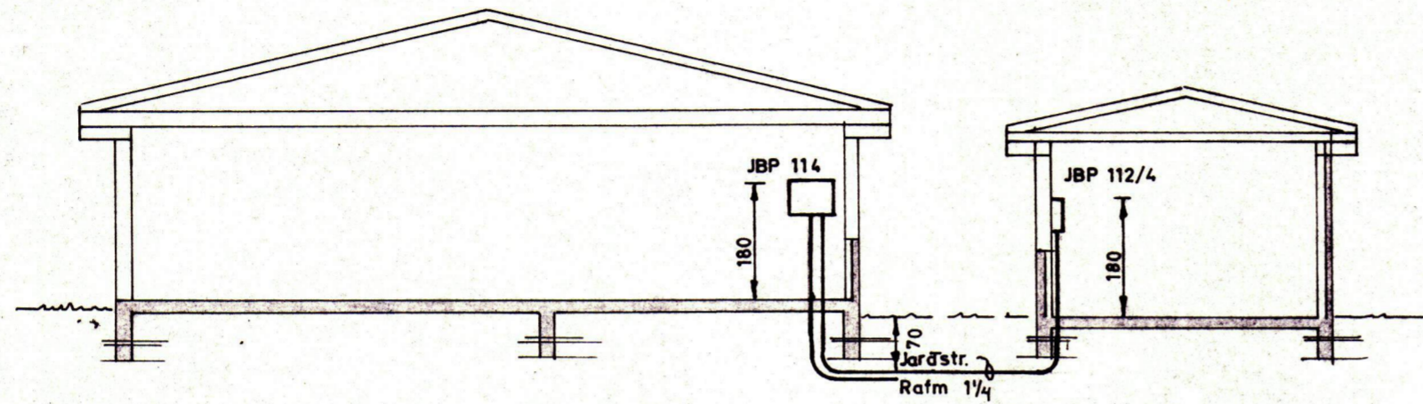
Snið M=1:100
