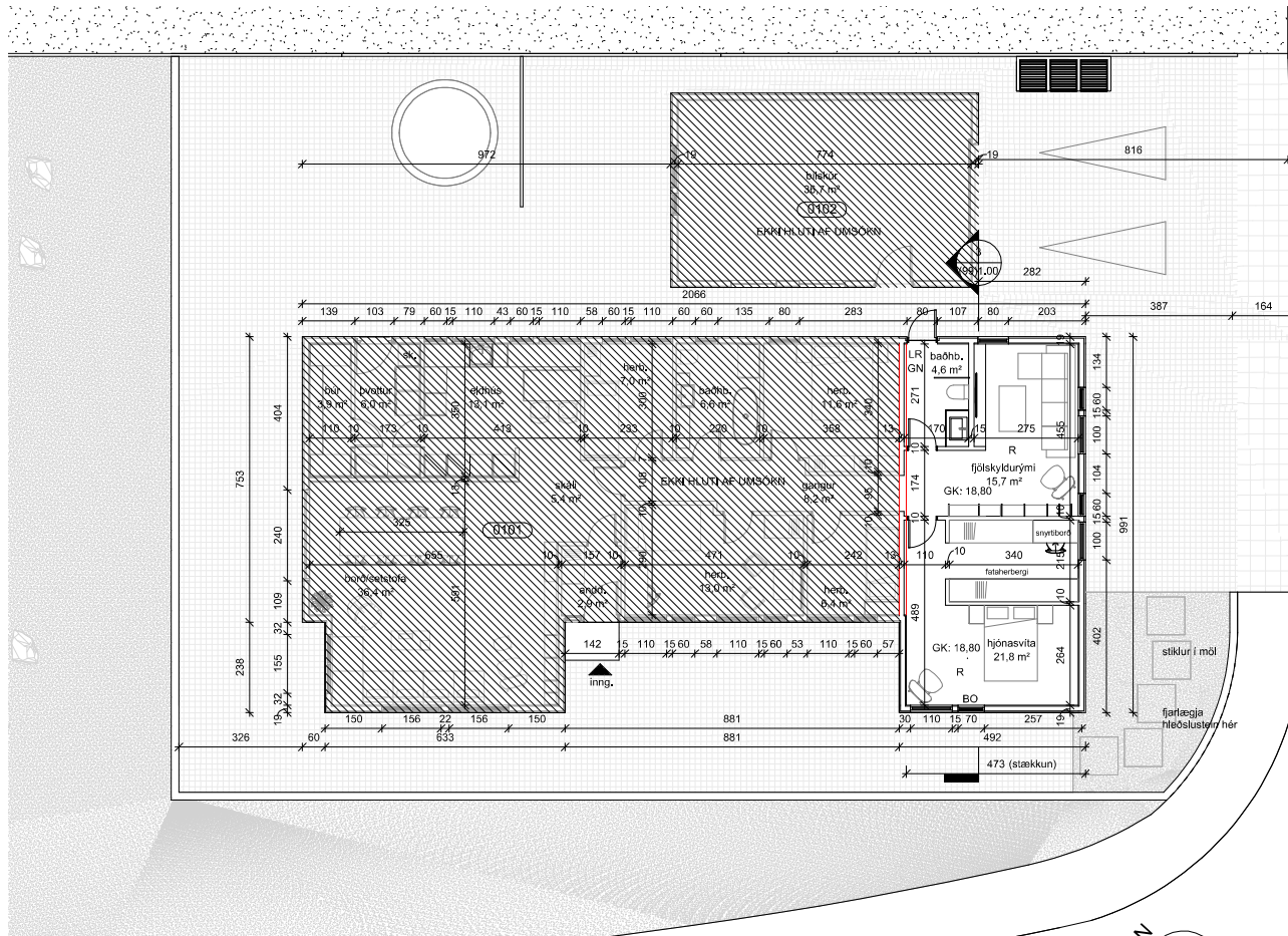
Grunnmynd 1 : 100
