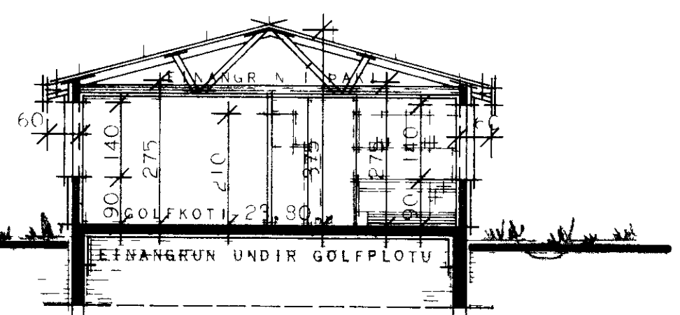
ÞVERSNEIÐING A-A
