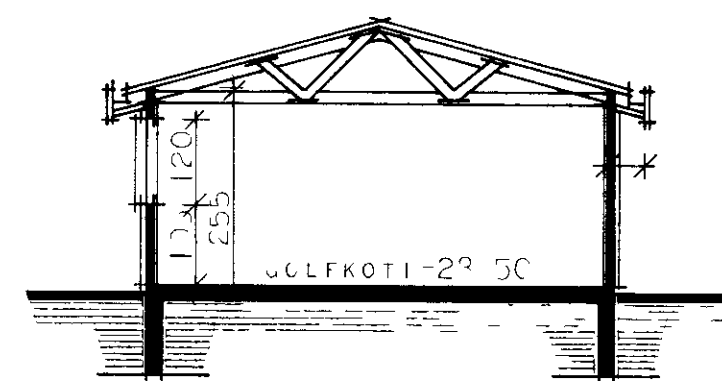
ÞVERSNEIÐING C-C
