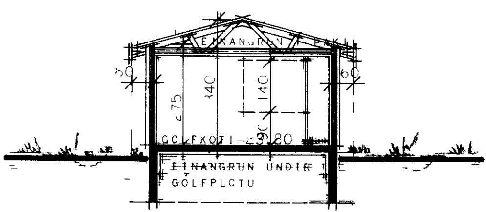
ÞVERSNEIÐING B-B
