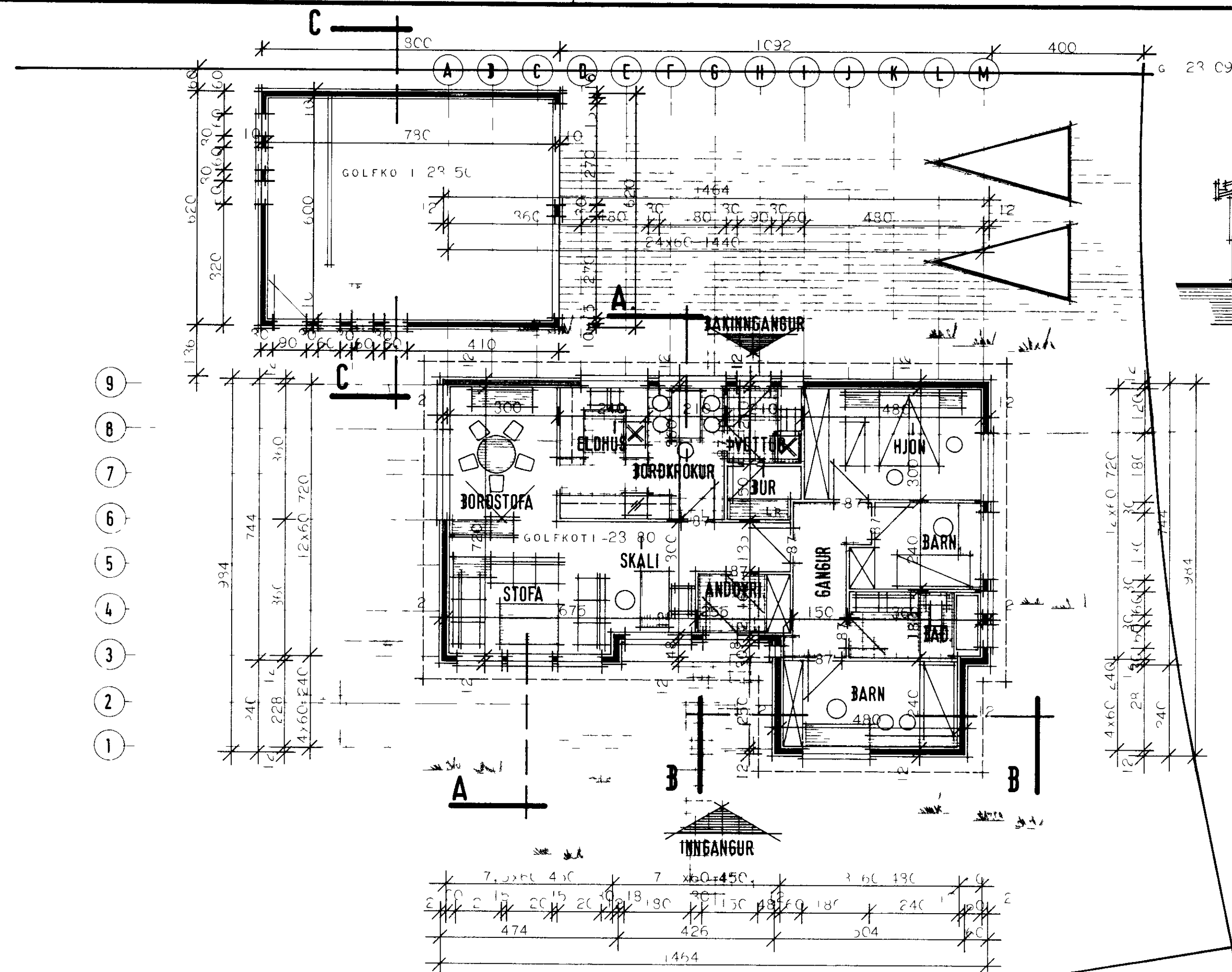
GRUNNMYND
