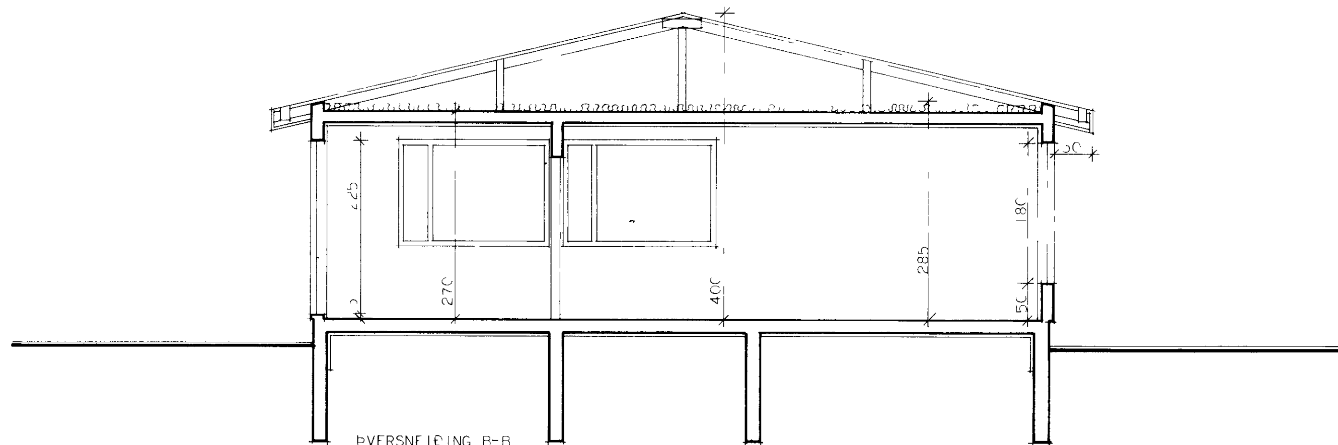
ÞVERSNEIÐING B-B
