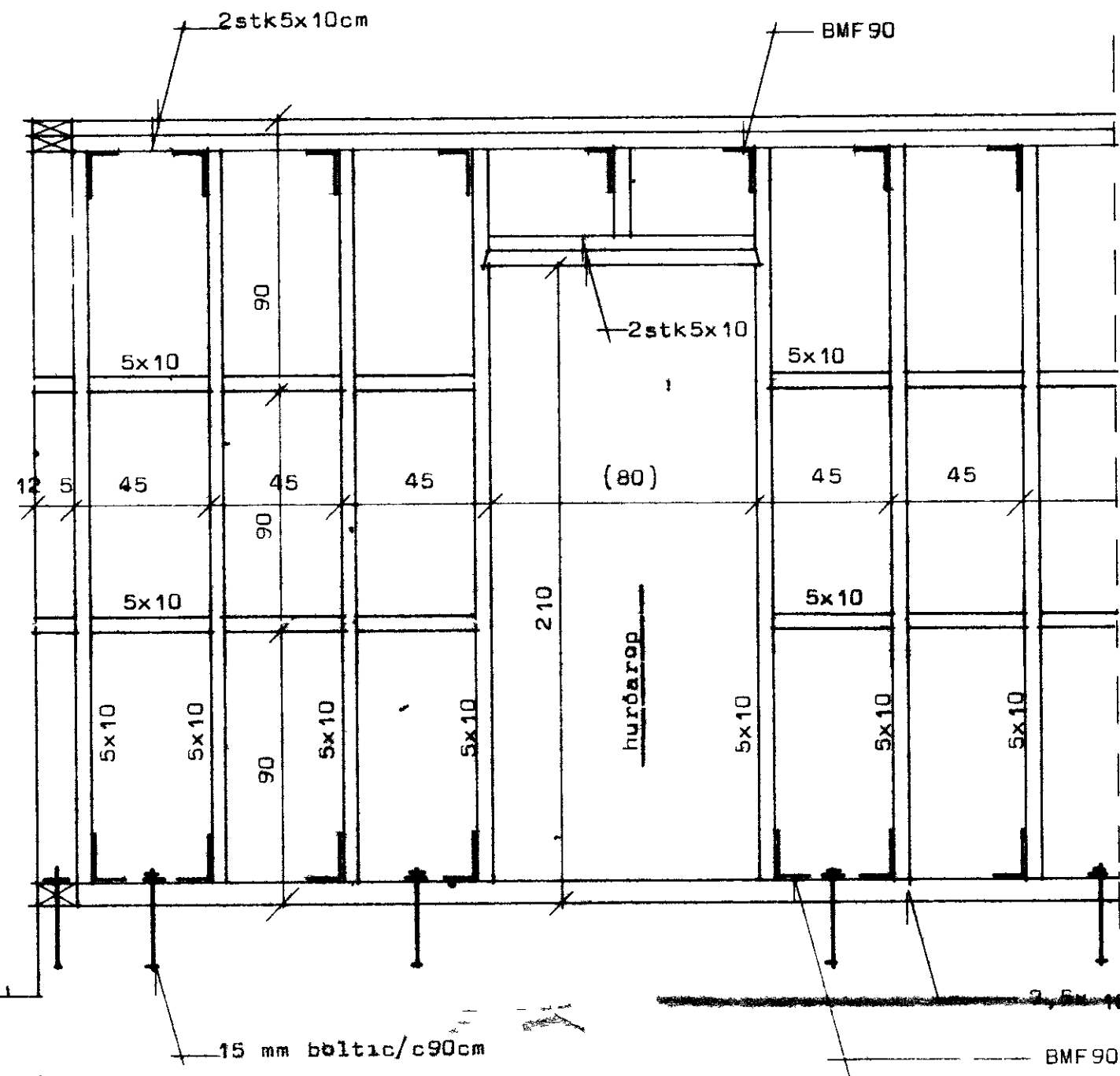
Fragangur a innvegg (burðarvegg)
