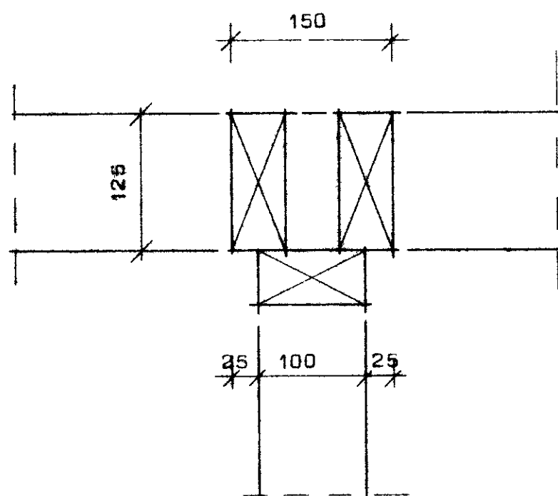
Fragangur a stoðum (innveggur að utvegg)
