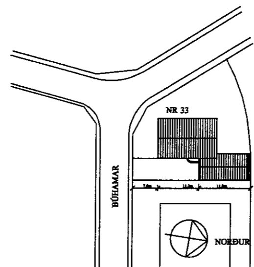
AFSTÖÐUMYND M=1 500
