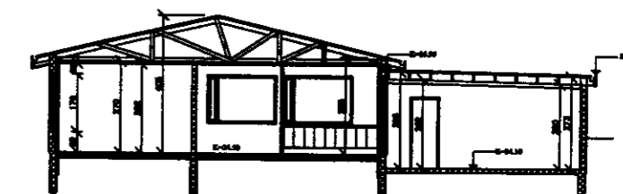
SNIÐ B-B
