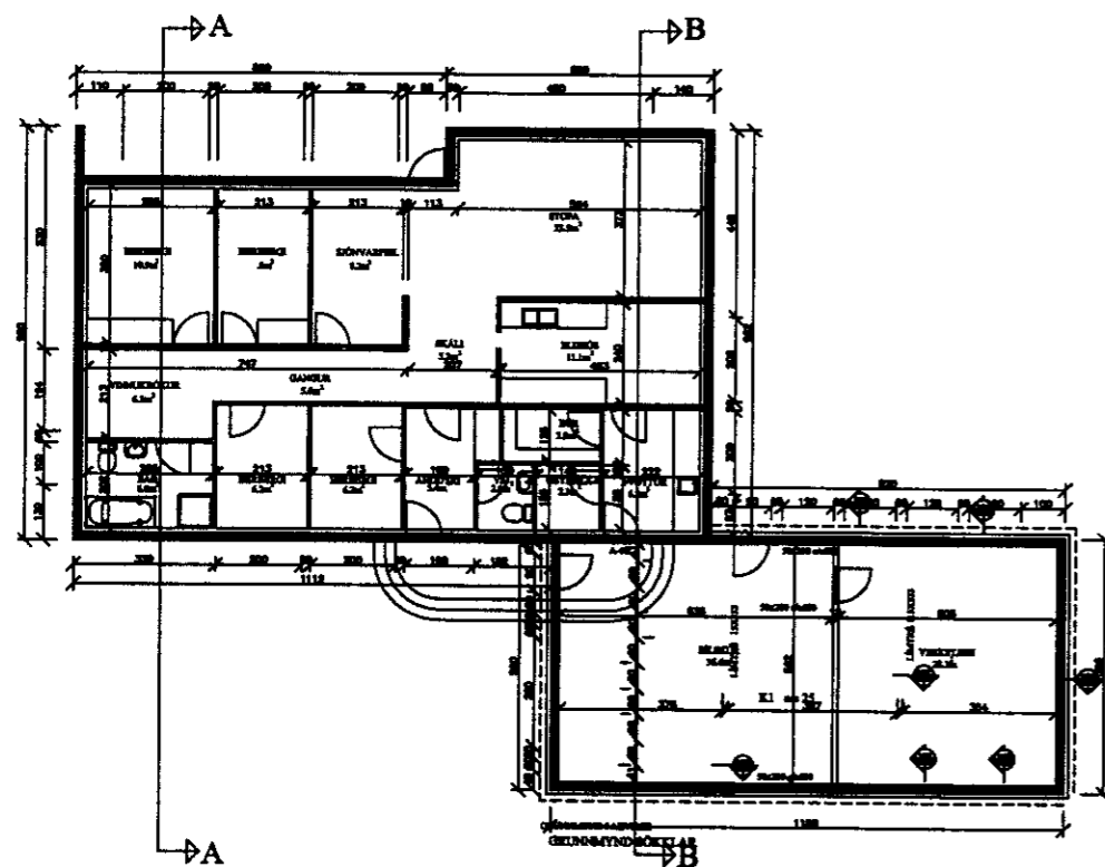
GRUNNMYND M=1 100
