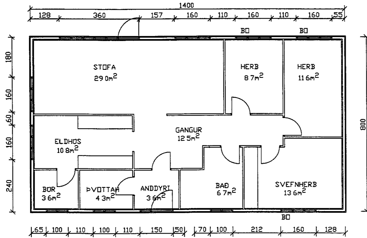
GRUNNMYND
