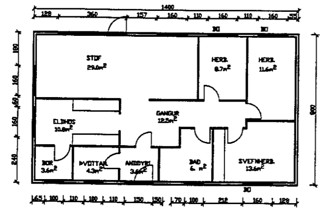
GRUNNMYND
